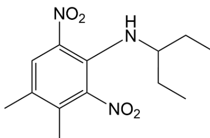
Obrázek 1: Strukturní vzorec pendimthalinu
