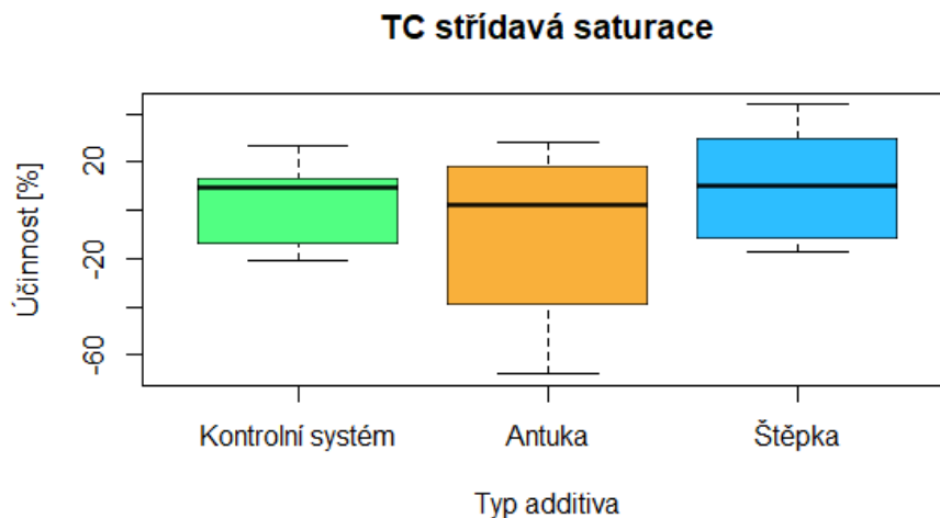
Graf č. 6 Celková účinnost filtračních materiálů při střídavé saturaci pro eliminaci celkového uhlíku
