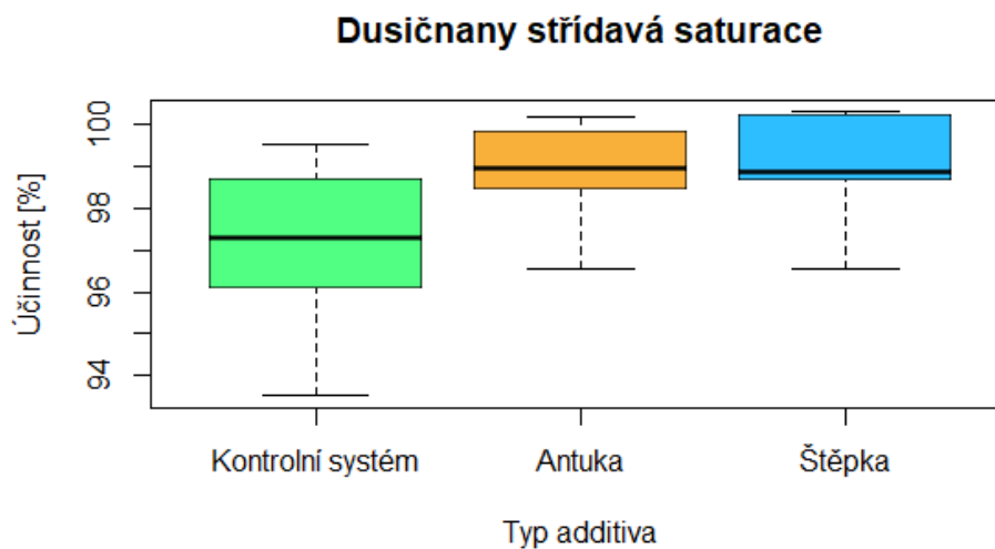
Graf č. 16 Celková účinnost filtračních materiálů při střídavé saturaci pro eliminaci dusičnan
