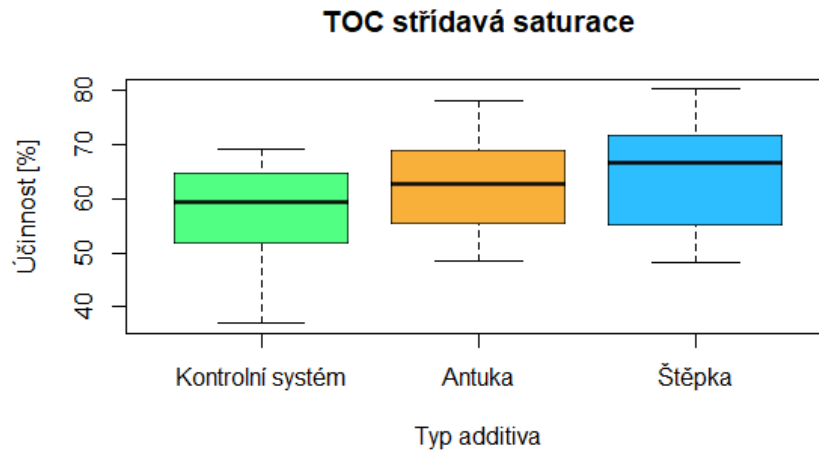
Graf č. 2 Celková účinnost filtračních materiálů při střídavé saturaci pro eliminaci celkového organického uhlíku
