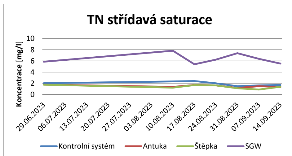
Graf č. 9 Celkový průběh koncentrace celkového dusíku při střídavé saturaci
