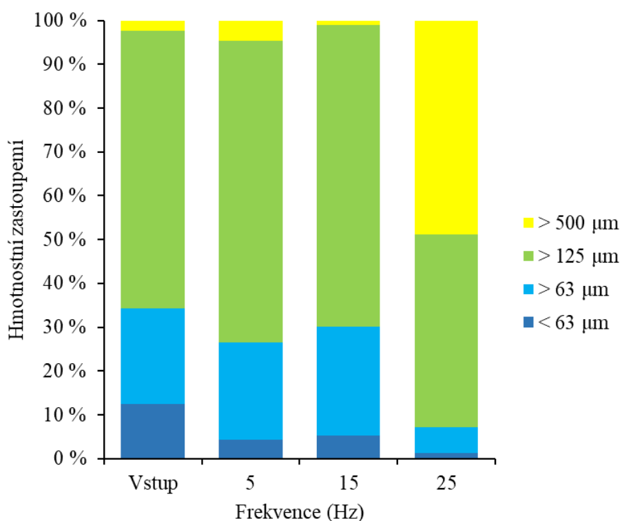
Obrázek 9: Hmotnostní zastoupení jednotlivých frakcí v závislosti na frekvenci mletí
