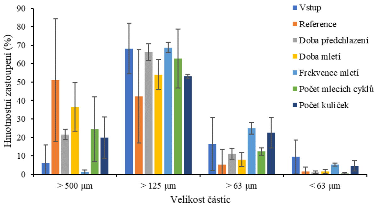
Obrázek 8: Graf procentuálního hmotnostního zastoupení velikostí jednotlivých přesetých frakcí
