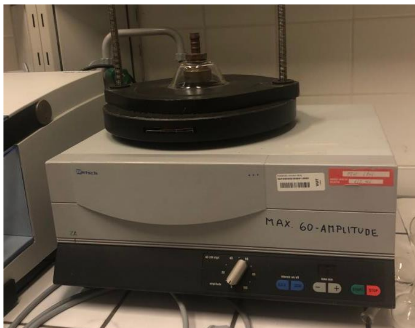
Obrázek 6: Laboratorní prosevačka Retsch AS 200 Digit
