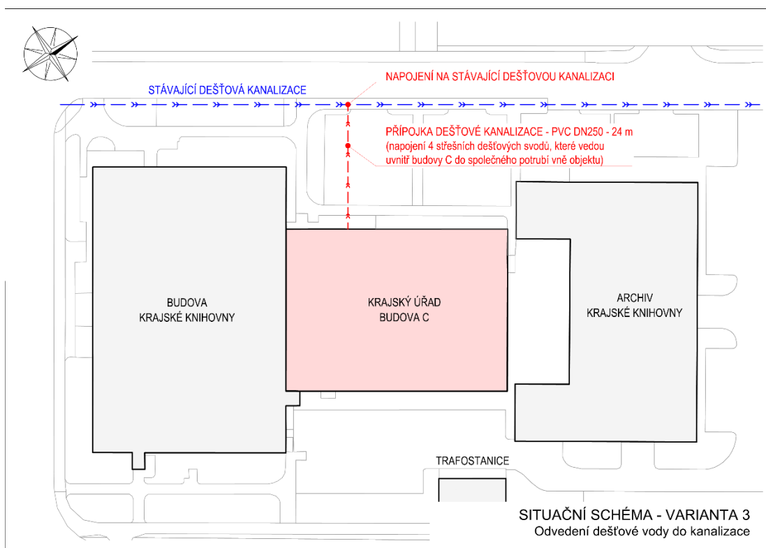
Obrázek 17: Situační schéma Varianta 3, Budova C (ČUZK, 2022)
