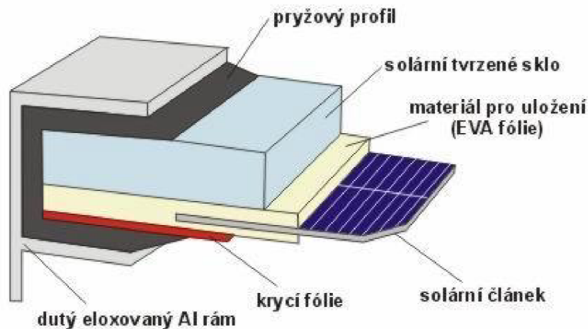
obr. 4 Řez fotovoltaickým panelem
