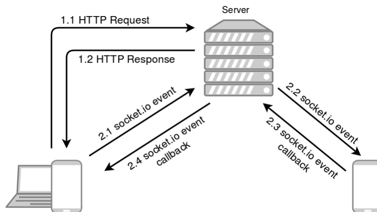
Obr. 5.1: Na obrázku je ukážka komunikácie aplikácie so serverom prostredníctvom HTTP a ukážka komunikácie medzi aplikáciami cez Socket.io.
