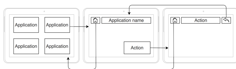
Obr. 5.7: Na obrázku je zobrazená zjednodušená navigácia v aplikácii pre seniora. Používateľ sa môže dostať maximálne do druhej úrovne zanorenia. Pokiaľ používateľ nie je na úvodnej obrazovke, je zobrazená horná lišta, ktorá vždy umožňuje návrat na úvodnú obrazovku alebo späť.
