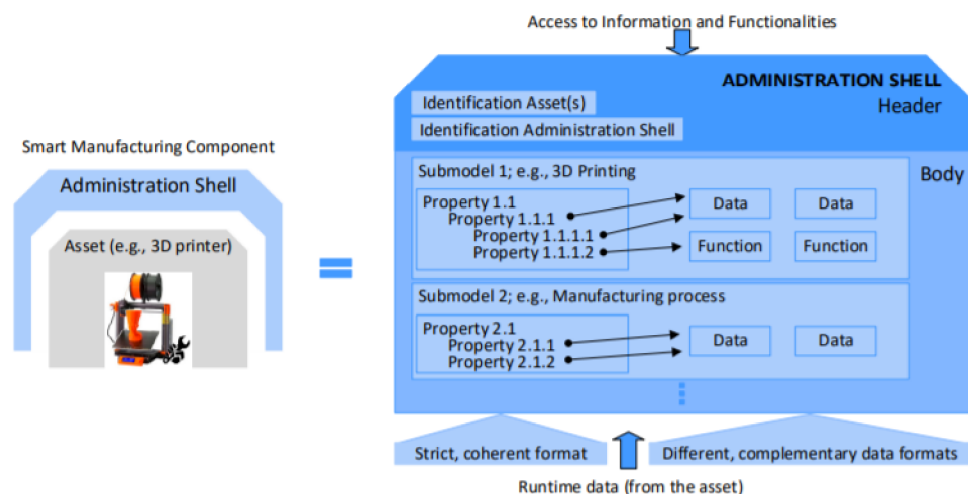
Obrázek 1.2 Struktura AAS [5]
