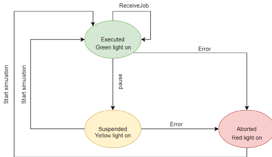
Obrázek 4.2 Stavů stanice
