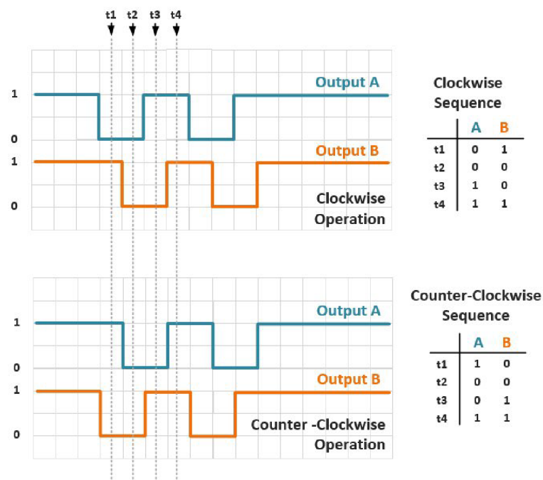
Obr. 2.1: Výstupy z kvadrurního enkodéru [9]
