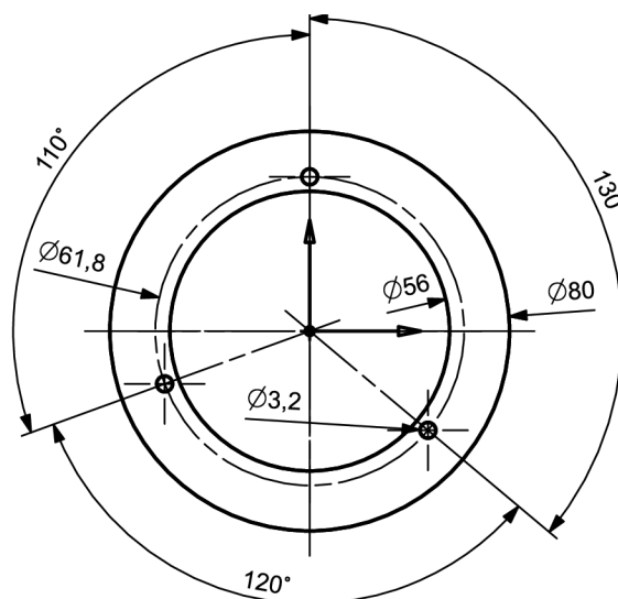
Obr. 6.3: Obecný náčrt kola pro první osu pouze s určujícími rozměry - za povšimnutí stojí nesymetrické umístění otvorů pro přichycení
