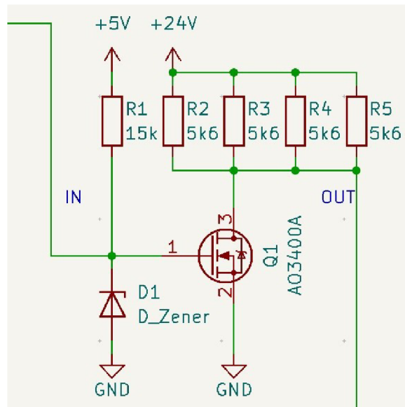
Obr. 6.7: Schéma jedné sekce level shifteru
