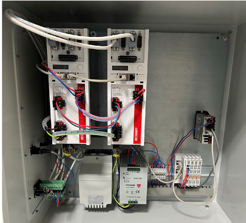
Obr. 4.4: Pohled na komponenty řídicího systému - Vlevo nahoře měniče, vedle měničů průmyslový počítač, pod měniči zleva snížovací transformátor pro motory, napájecí zdroj 24VDC a coupler v němž jsou zasunuty vstupní a výstupní karty
