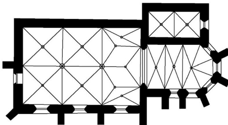
30. Soběslav, kostel sv. Víta, půdorys, třetí čtvrtina 14. století.
