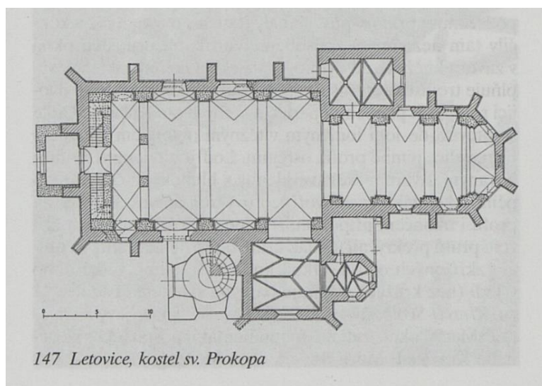
6. Letovice, kostel sv. Prokopa, půdorys, poslední čtvrtina 14. století.
