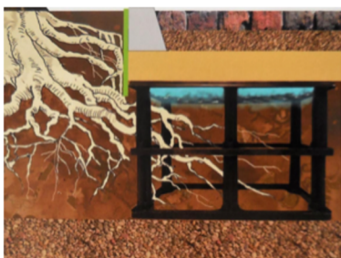
Obr. XVII. Prokořenitelné zemní buňky TreeParker (zdroj: bluegreen.com )
