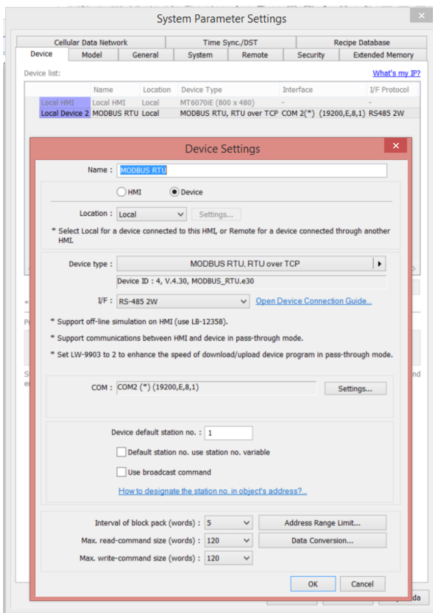
Obr. 4.1: Nastavení pro Modbus RTU
