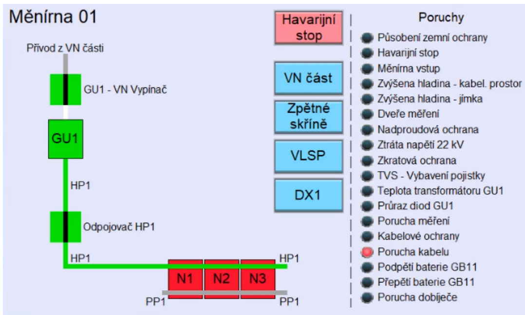
Obr. 4.3: Přehled měničny na HMI panelu
