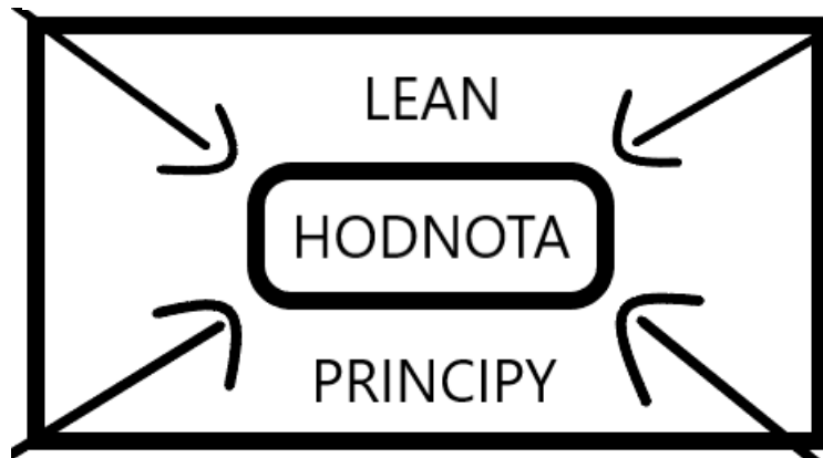
Obrázek 1: lean principy
