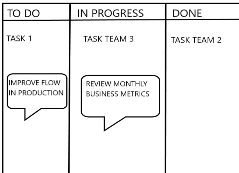
Obrázek 2: Kanbanová deska
