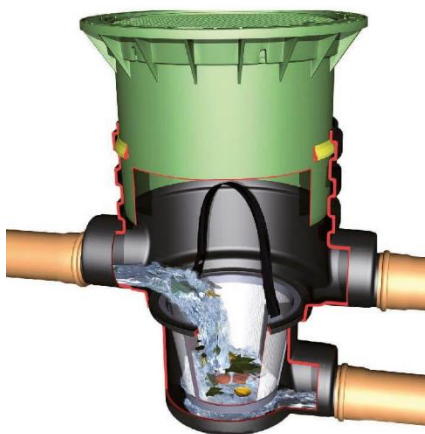
Obrázek 13: Detail filtrační šachty DN400 s vyjímatelným košíkem
