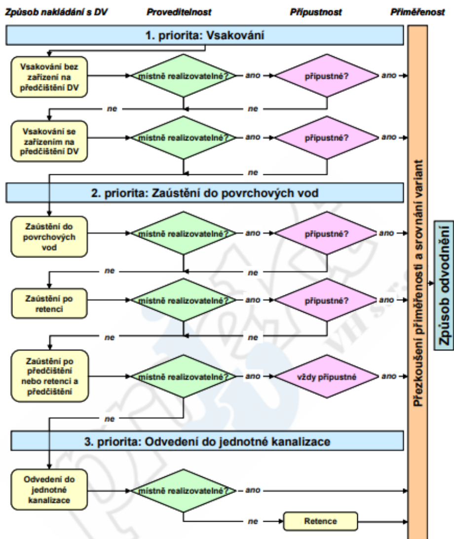
Obrázek 5 – Priority nakládání s dešťovými vodami a volba způsobu odvodnění
