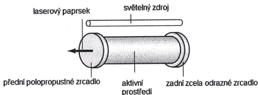
Obr. 4 Schéma rezonátoru [3].
