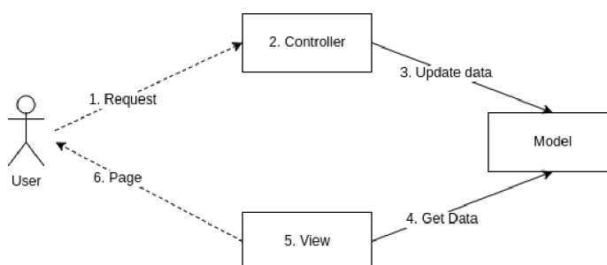
Obrázek 5.1: Architektura MVC
