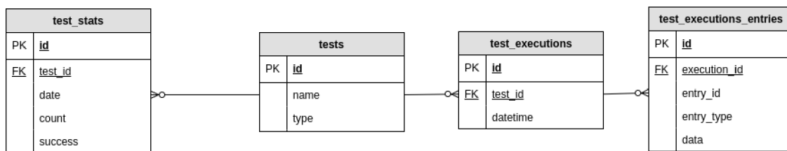
Obrázek 5.3: ER diagram
