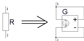
Obr. 6.1: Náhradní schéma zapojení odporu ideálním zdrojem proudu řízeného napětím.
