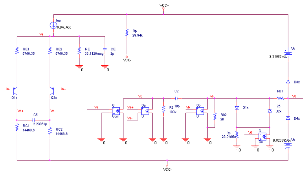
Obr. 3.4: Schéma zapojení navrženého modelu v programu OrCAD PSpice.
