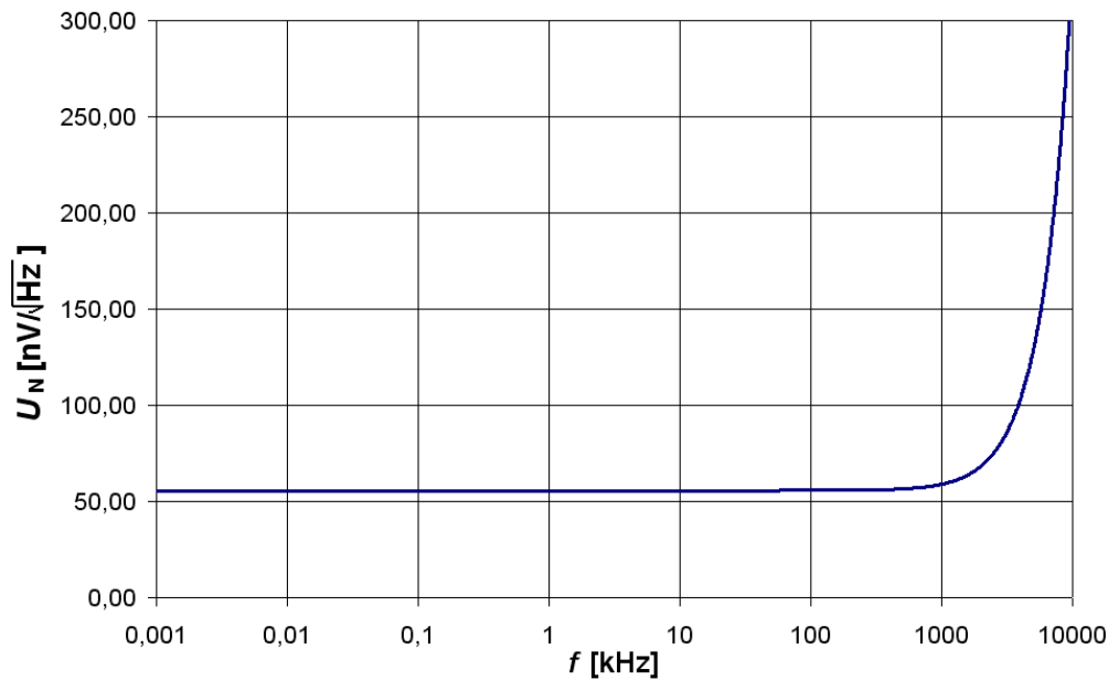
Obr. 6.4: Simulace vstupního šumového napětí pro navržený makromodel.
