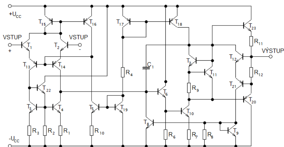
Obr. 1.6: Model (mikromodel) 6. úrovně operačního zesilovače LM741 (převzato [6]).
