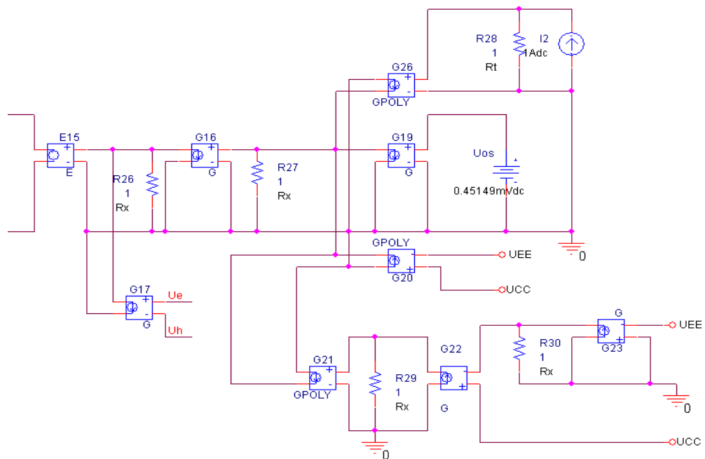
Obr. 8.5: Schéma zapojení řízených zdrojů pro nastavení zbytkového napětí OZ.
