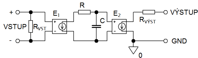
Obr. 1.3: Lineární dynamický jednopólový model 3. úrovně reálného OZ (převzato z [6]).
