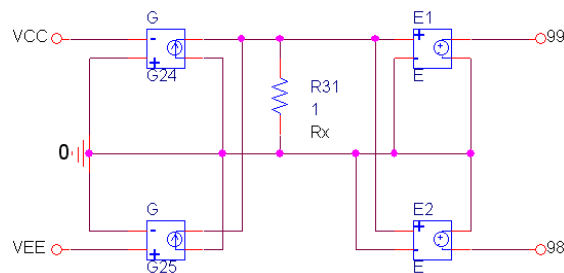
Obr. 8.6: Schéma zapojení pro převedení nesymetrického napětí na symetrické.
