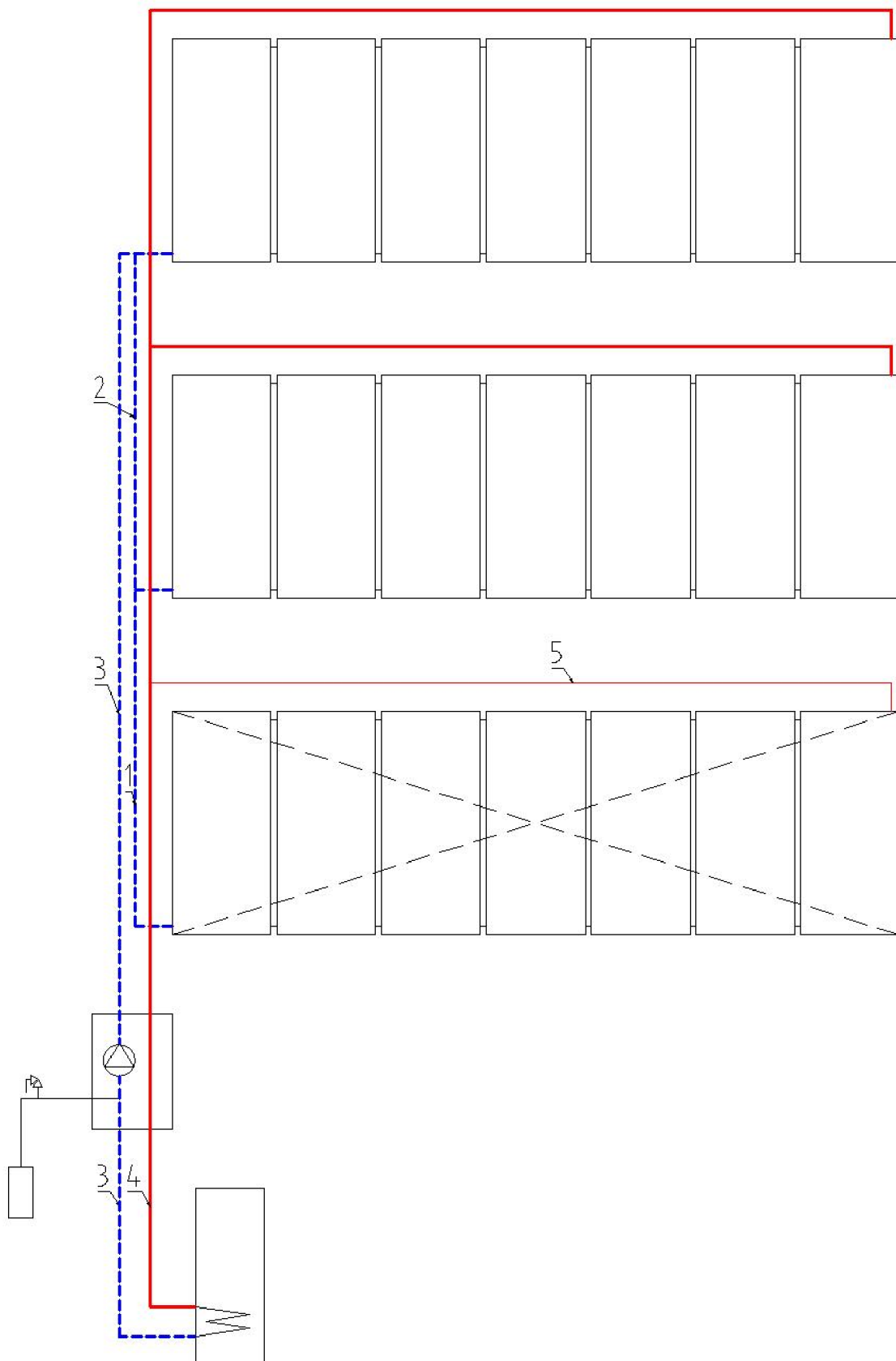
Obrázok 13 Dimenzačná schéma solárnych kolektorov
