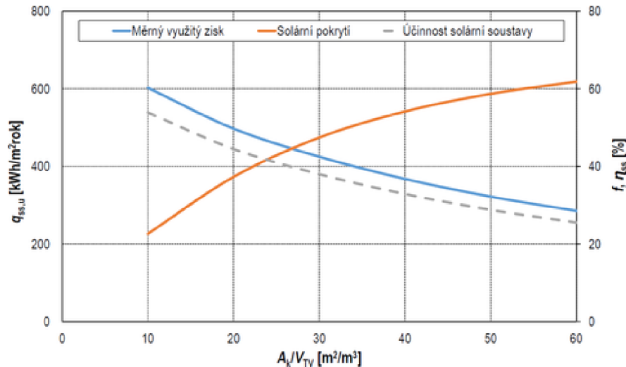
Obrázok 9 Vplyv pomeru plochy kolektoru k dennej spotrebe vody na celkovej bilancií systému [21]
