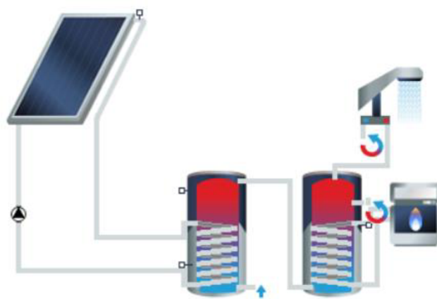
Obrázok 15 Schematické zapojenie zásobníkov, model T*sol [31]
