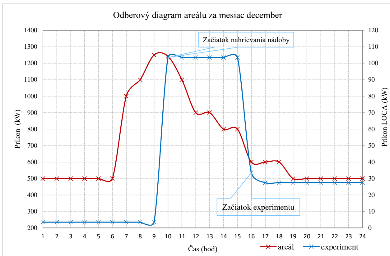
Obr. 14 Optimalizácia zariadenia LOCA v mesiaci december
