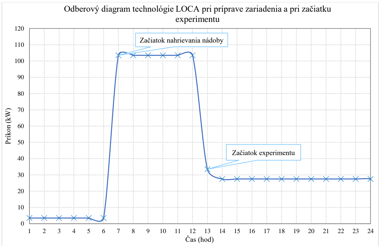
Obr. 12 Odberový diagram zariadenia LOCA
