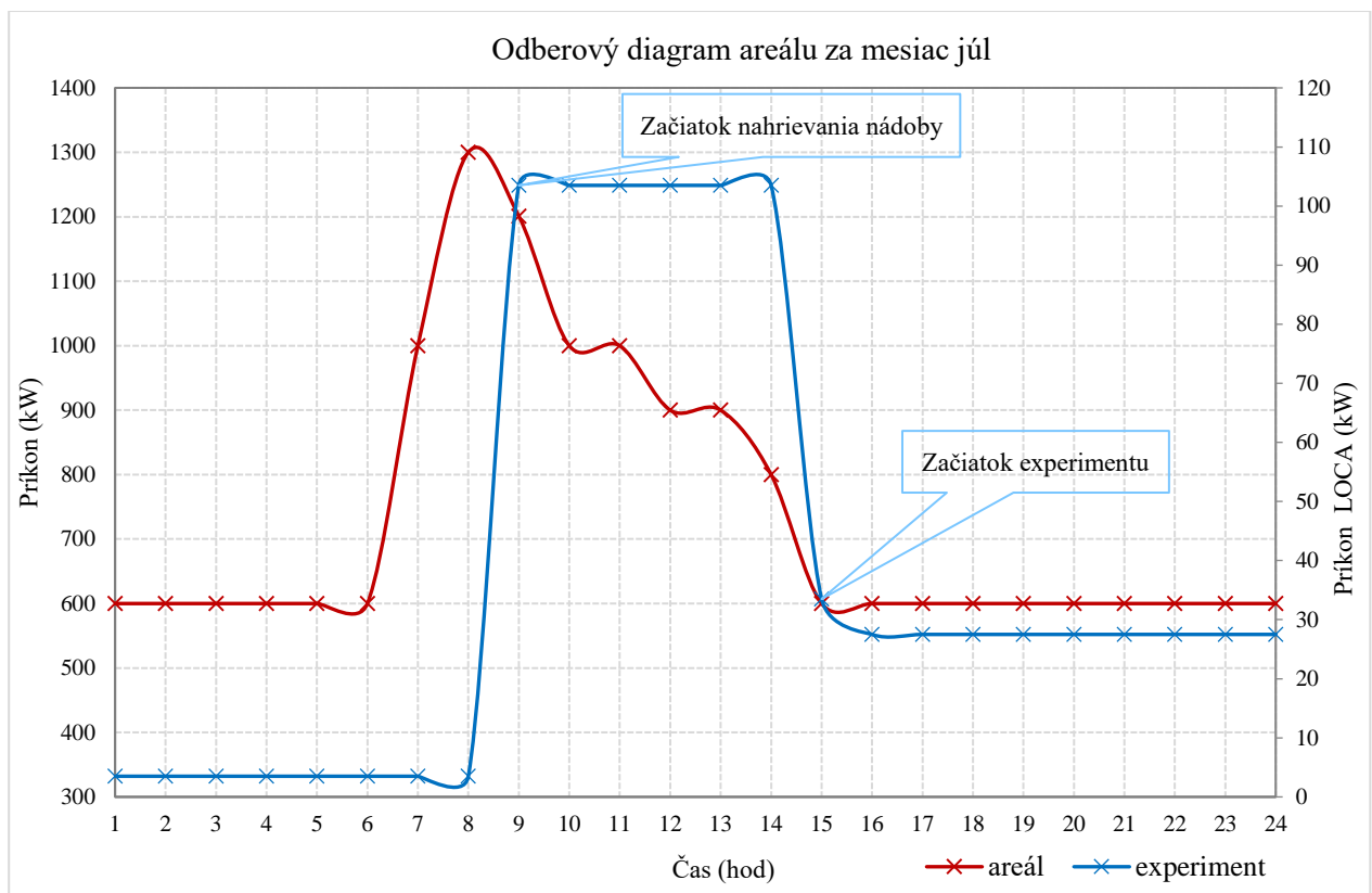
Obr. 13 Optimalizácia zariadenia LOCA v mesiaci júl
