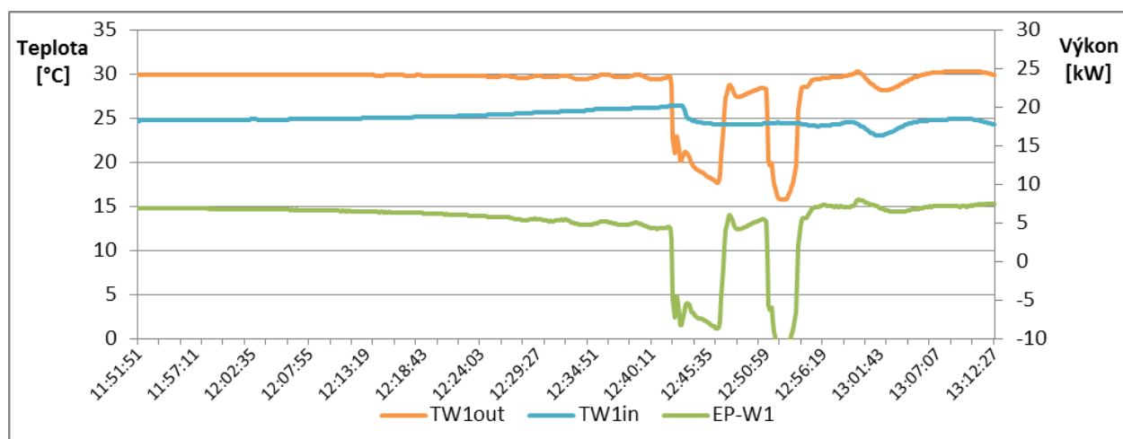
Obr. 39 Zdvojený odtávací cyklus
