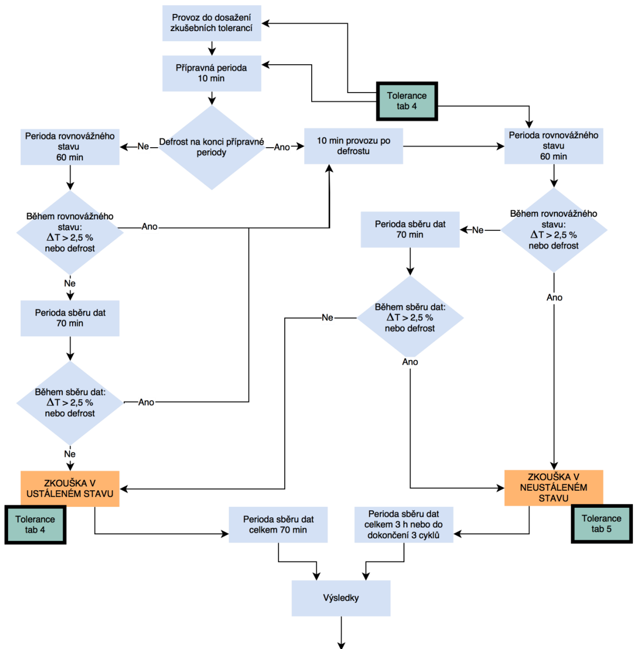
Obr. 11 Zkušební postup
