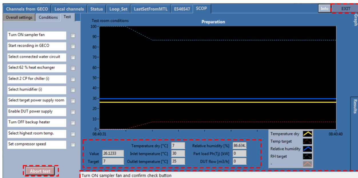
Obr. 17 Rozložení a další funkce
