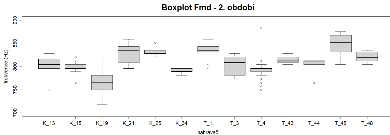
Obrázek 23. Variabilita hodnot mezi jedinci (nahrávači) pro parametr Fmd, zaznamenaných během 2. nahrávacího období roku 2015 v Krušných horách a na Třeboňsku. Zobrazen je medián, minimum, maximum, 25% a 75% kvartily a odlehlé hodnoty pro individuální jedince.
