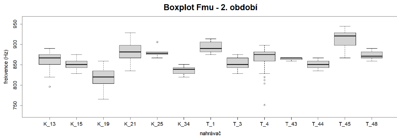
Obrázek 24. Variabilita hodnot mezi jedinci (nahrávači) pro parametr Fmu, zaznamenaných během 2. nahrávacího období roku 2015 v Krušných horách a na Třeboňsku. Zobrazen je medián, minimum, maximum, 25% a 75% kvartily a odlehlé hodnoty pro individuální jedince.
