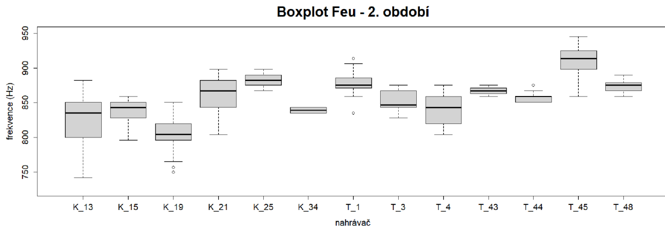
Obrázek 26. Variabilita hodnot mezi jedinci (nahrávači) pro parametr Feu, zaznamenaných během 2. nahrávacího období roku 2015 v Krušných horách a na Třeboňsku. Zobrazen je medián, minimum, maximum, 25% a 75% kvartily a odlehle hodnoty pro individuální jedince.
