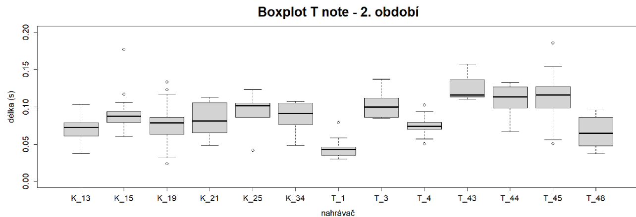
Obrázek 28. Variabilita hodnot mezi jedinci (nahrávači) pro parametr T note, zaznamenaných během 2. nahrávacího období roku 2015 v Krušných horách a na Třeboňsku. Zobrazen je medián, minimum, maximum, 25% a 75% kvartily a odlehle hodnoty pro individuální jedince.
