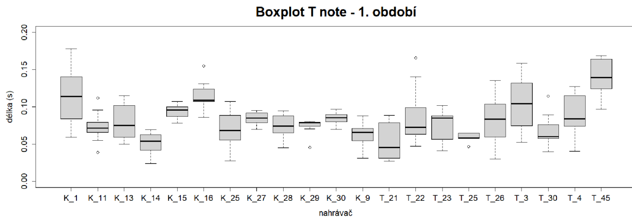
Obrázek 19. Variabilita hodnot mezi jedinci (nahrávači) pro parametr T note zaznamenaných během 1. nahrávacího období roku 2015 v Krušných horách a na Třeboňsku. Zobrazen je medián, minimum, maximum, 25% a 75% kvartily a odlehle hodnoty pro individuální jedince.
