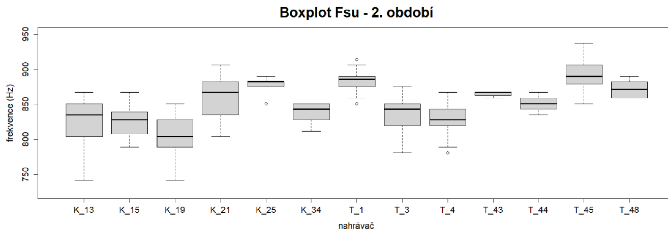
Obrázek 22. Variabilita hodnot mezi jedinci (nadržávači) pro parametr Fsu, zaznamenaných během 2. nadržovacího období roku 2015 v Krušných horách a na Třeboňsku. Zobrazen je medián, minimum, maximum, 25% a 75% kvartily a odlehlé hodnoty pro individuální jedince.
