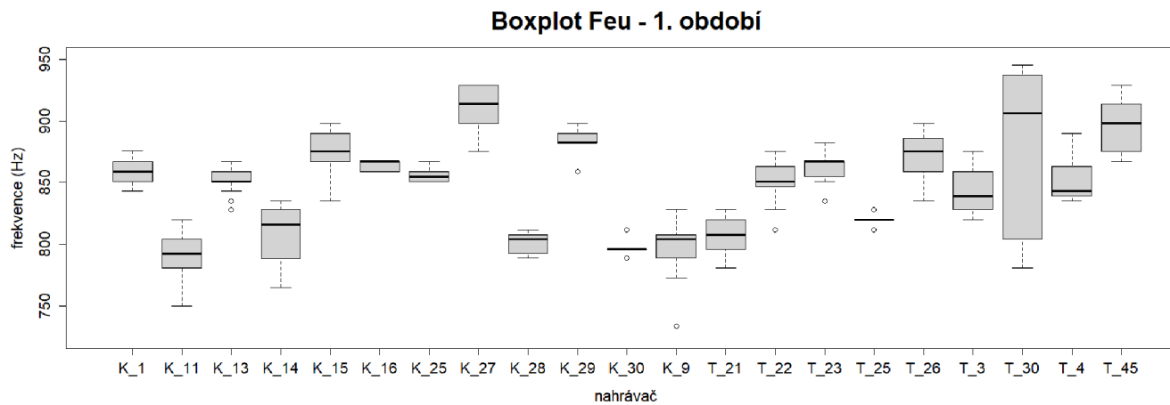
Obrázek 17. Variabilita hodnot mezi jedinci (nahrávači) pro parametr Feu zaznamenaných během 1. nahrávacího období roku 2015 v Krušných horách a na Třeboňsku. Zobrazen je medián, minimum, maximum, 25% a 75% kvartily a odlehlé hodnoty pro individuální jedince.
