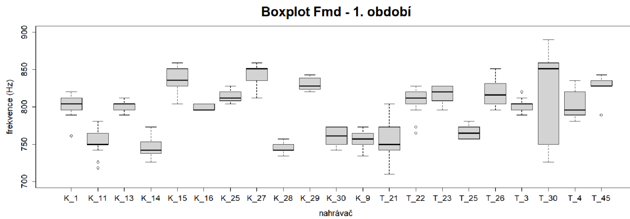
Obrázek 14. Variabilita hodnot mezi jedinci (nahrávači) pro parametr Fmd zaznamenaných během 1. nahrávacího období roku 2015 v Krušných horách a na Třebořsku. Zobrazen je medián, minimum, maximum, 25% a 75% kvartily a odlehlé hodnoty pro individuální jedince.
