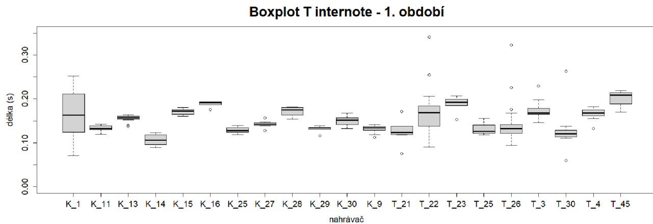
Obrázek 20. Variabilita hodnot mezi jedinci (nahrávači) pro parametr T internote zaznamenaných během 1. nahrávacího období roku 2015 v Krušných horách a na Třeboňsku. V rámci boxplotu je zobrazen medián, minimum, maximum, 25% a 75% kvartily a odlehle hodnoty pro individuální jedince.
