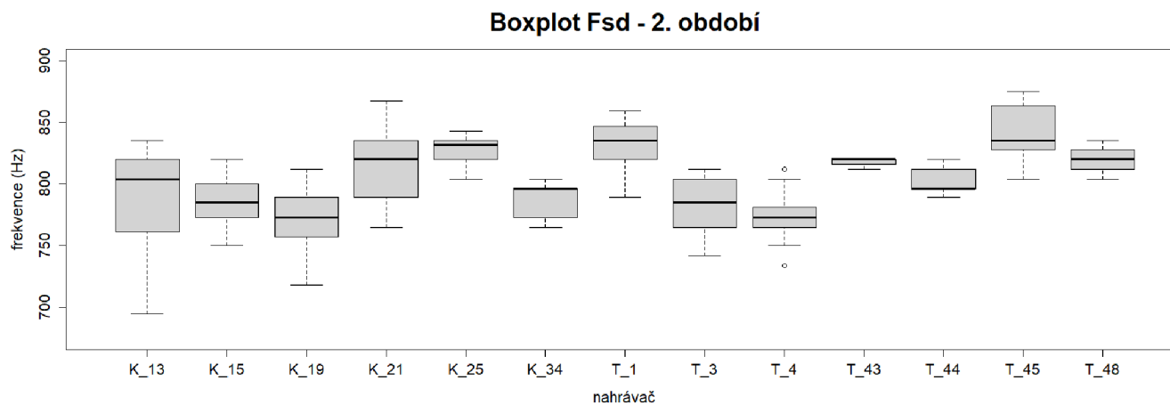
Obrázek 21. Variabilita hodnot mezi jedinci (nahrávači) pro parametr Fsd, zaznamenaných během 2. nadržovacího období roku 2015 v Krušných horách a na Třeboňsku. Zobrazen je medián, minimum, maximum, 25% a 75% kvartily a odlehlé hodnoty pro individuální jedince.
