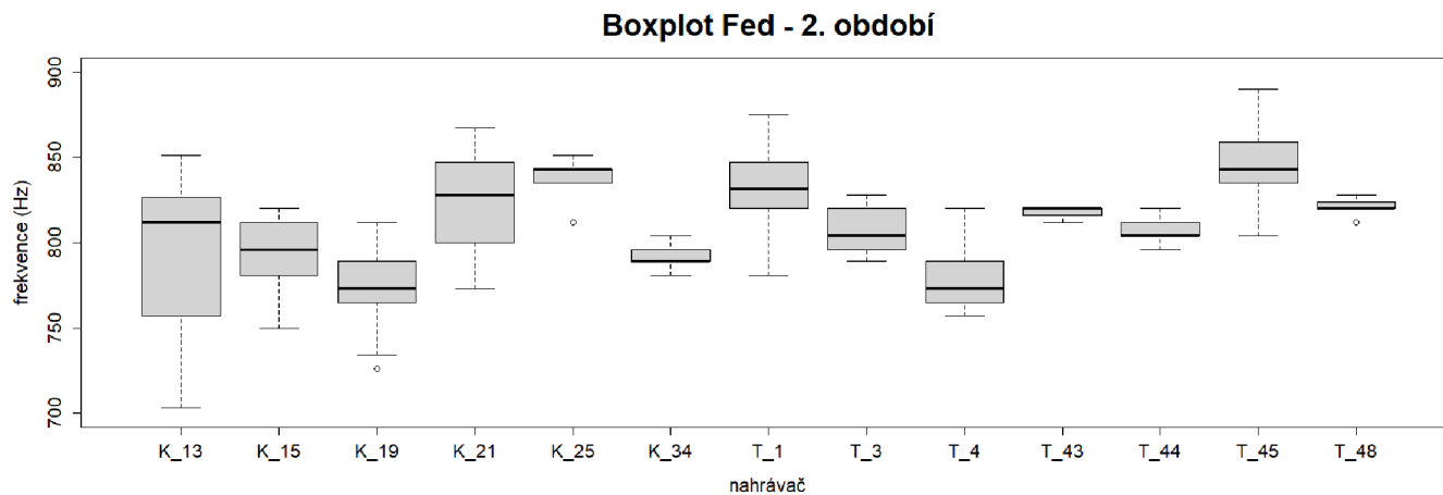
Obrázek 25. Variabilita hodnot mezi jedinci (nahrávači) pro parametr Fed, zaznamenaných během 2. nahrávacího období roku 2015 v Krušných horách a na Třeboňsku. Zobrazen je medián, minimum, maximum, 25% a 75% kvartily a odlehle hodnoty pro individuální jedince.
