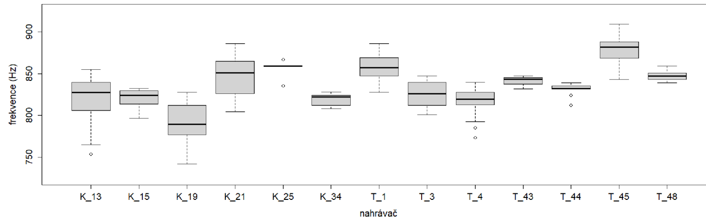
Obrázek 27. Variabilita hodnot mezi jedinci (nahrávači) pro parametr Fi, zaznamenaných během 2. nahrávacího období roku 2015 v Krušných horách a na Třeboňsku. Zobrazen je medián, minimum, maximum, 25% a 75% kvartily a odlehlé hodnoty pro individuální jedince.
