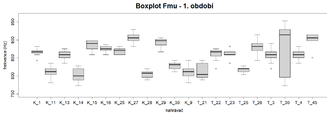
Obrázek 15. Variabilita hodnot mezi jedinci (nahrávači) pro parametr Fmu zaznamenaných během 1. nahrávacího období roku 2015 v Krušných horách a na Třebořsku. Zobrazen je medián, minimum, maximum, 25% a 75% kvartily a odlehlé hodnoty pro individuální jedince.
