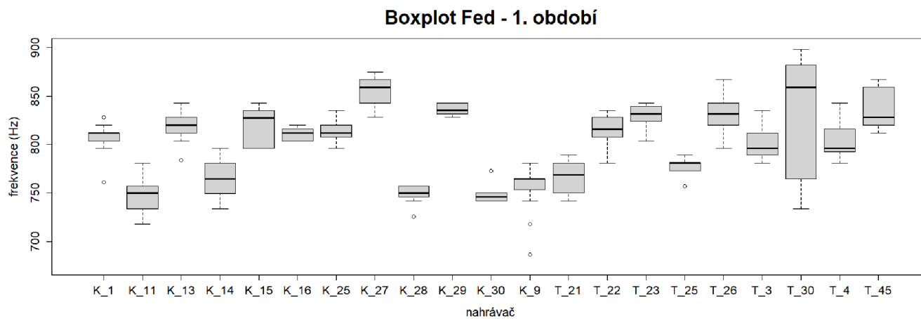
Obrázek 16. Variabilita hodnot mezi jedinci (nahrávači) pro parametr Fed zaznamenaných během 1. nahrávacího období roku 2015 v Krušných horách a na Třeboňsku. Zobrazen je medián, minimum, maximum, 25% a 75% kvartily a odlehlé hodnoty pro individuální jedince.
