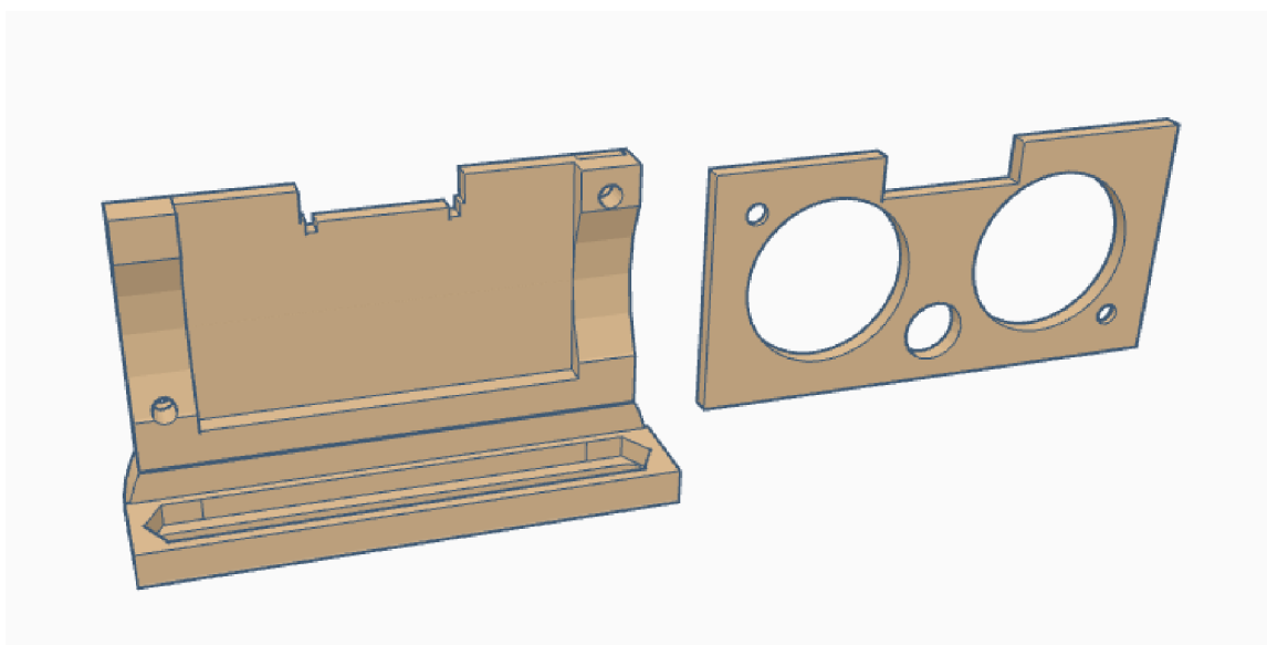
Obrázek A.2: Adaptér na senzory vzdálenosti SRF-08. Lze přitom použít bez části vpravo, která má chránit samotný tištěný spoj. Jelikož byly otvory pro uchycení adaptérů vrtány ručně s poměrně velkou tolerancí vůči nepřesnostem, umožňuje sonar variabilní rozstup montážních otvorů (místo dvou otvorů pro šrouby je v dolní části podlouhlý otvor pro libovolné umístění šroubů).
