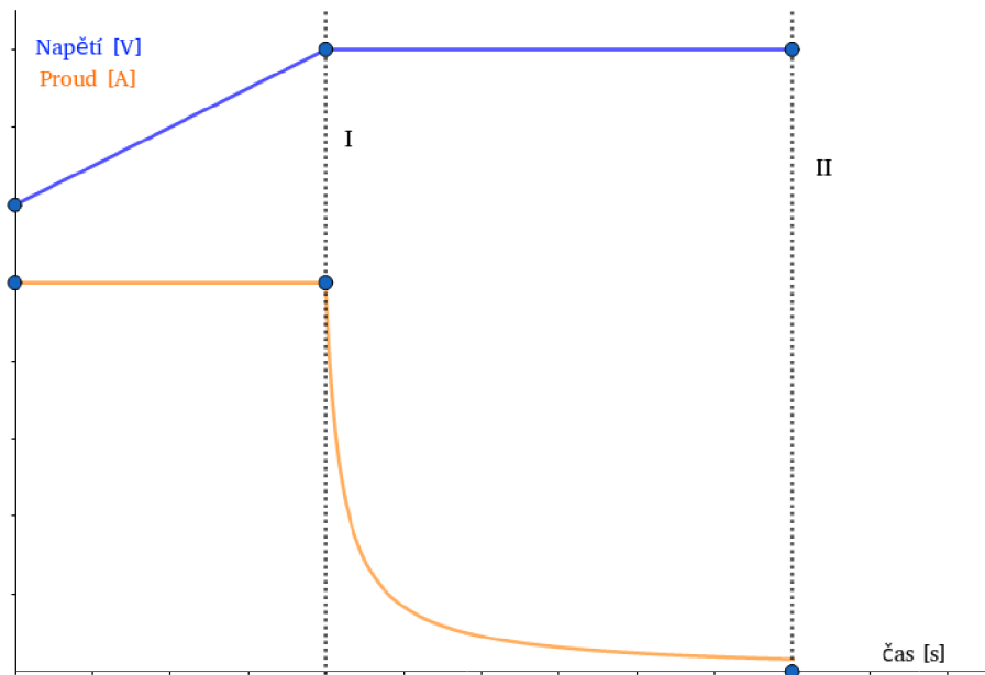
Obrázek 3.1: Ilustrační graf nabíjení metodou CC/CV. Od počátku grafu do svislé tečkované přímky označené jako I probíhá fáze CC (z angl. constant current ), poté do přímky II probíhá fáze CV ( constant voltage ). Následně je již proud tak malý, že je nabíjení ukončeno. Osy grafu jsou úmyslně nepopsány, vzhledem k tomu, že konkrétní hodnoty se liší podle typu baterie, požadavků na rychlost nabíjení atp.
