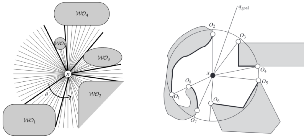
Obrázek 2.4: Ukázka bodu nespojitosti a intervalů kontinuity (například tučně vyznačený interval mezi body O_3 a O_4 ). Obrázek přejet z [11].
