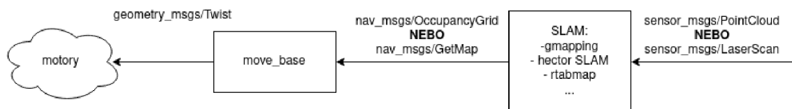
Obrázek 7.4: Minimalistické schéma jádra ovládacího programu pro mobilního robota v ROS.
