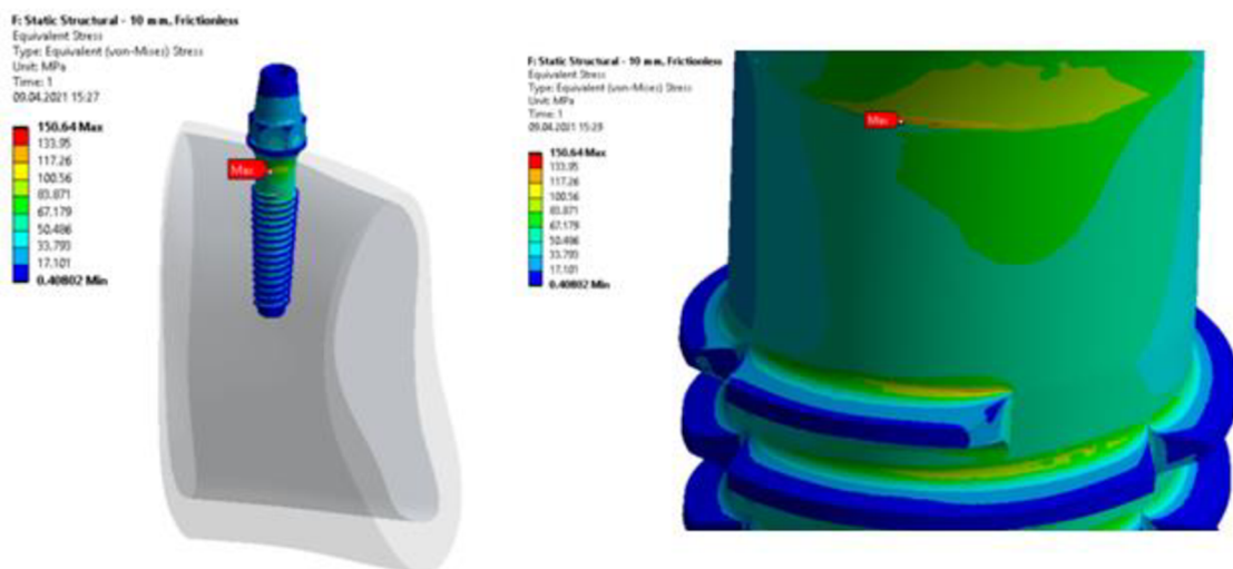
Obrázek 28 - Výsledky redukováného napětí implantátu A10 nepřirostlé kortiky
