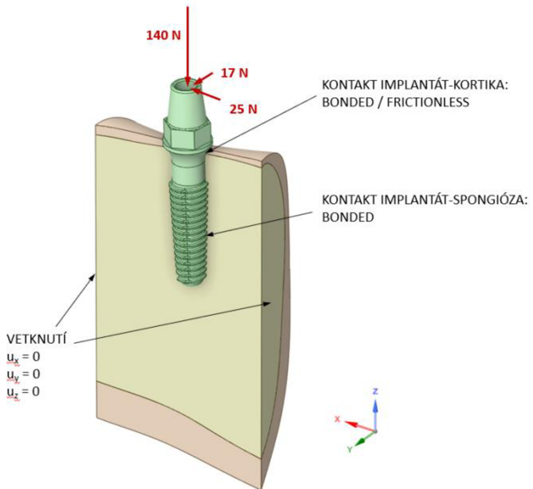
Obrázek 26 - Okrajové podmínky
