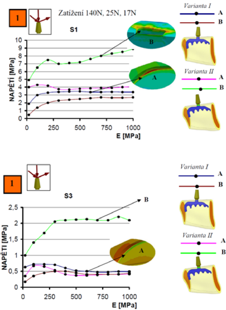
Obrázek 36 - Výsledky hlavního napětí pro modul pružnosti 1000 MPa srovnávané s diplomovou prací Mgr. Petrlíkové
