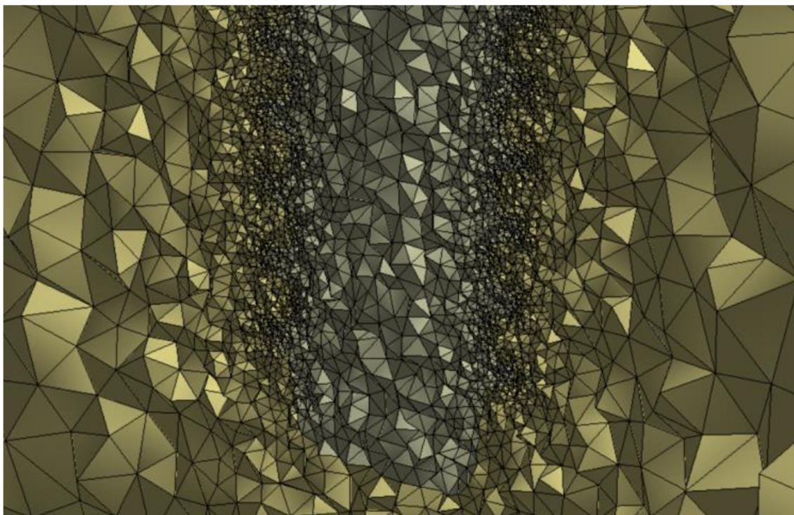
Obrázek 24 - Detail sítě
