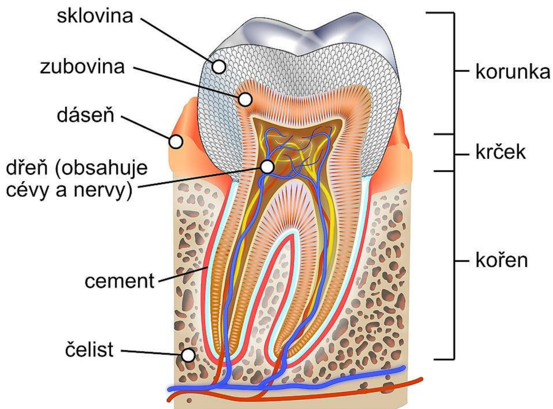
Obrázek 8 - Stavba zubu [5]
