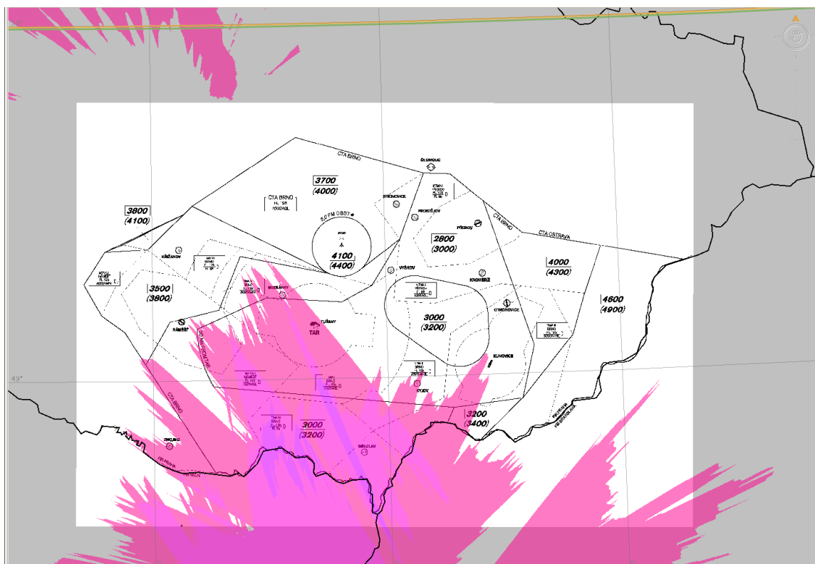
Obr. 19 Pokrytí sekundárními radary v okolí LKTB ve výšce 1500 ft AGL, vytvořeno v EUROCONTROL SASS-C PREDICtION/CAPT 2.2.6, publikováno se souhlasem ŘLP ČR s.p.
