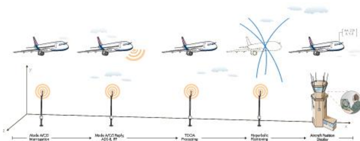
Obr. 9 Princip funkce multilaterace [11]
