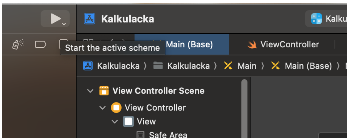
Obrázek 16 - zapínání simulace
