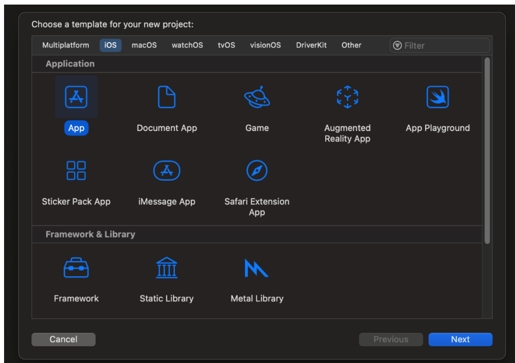
Obrázek 6 - výběr platformy
