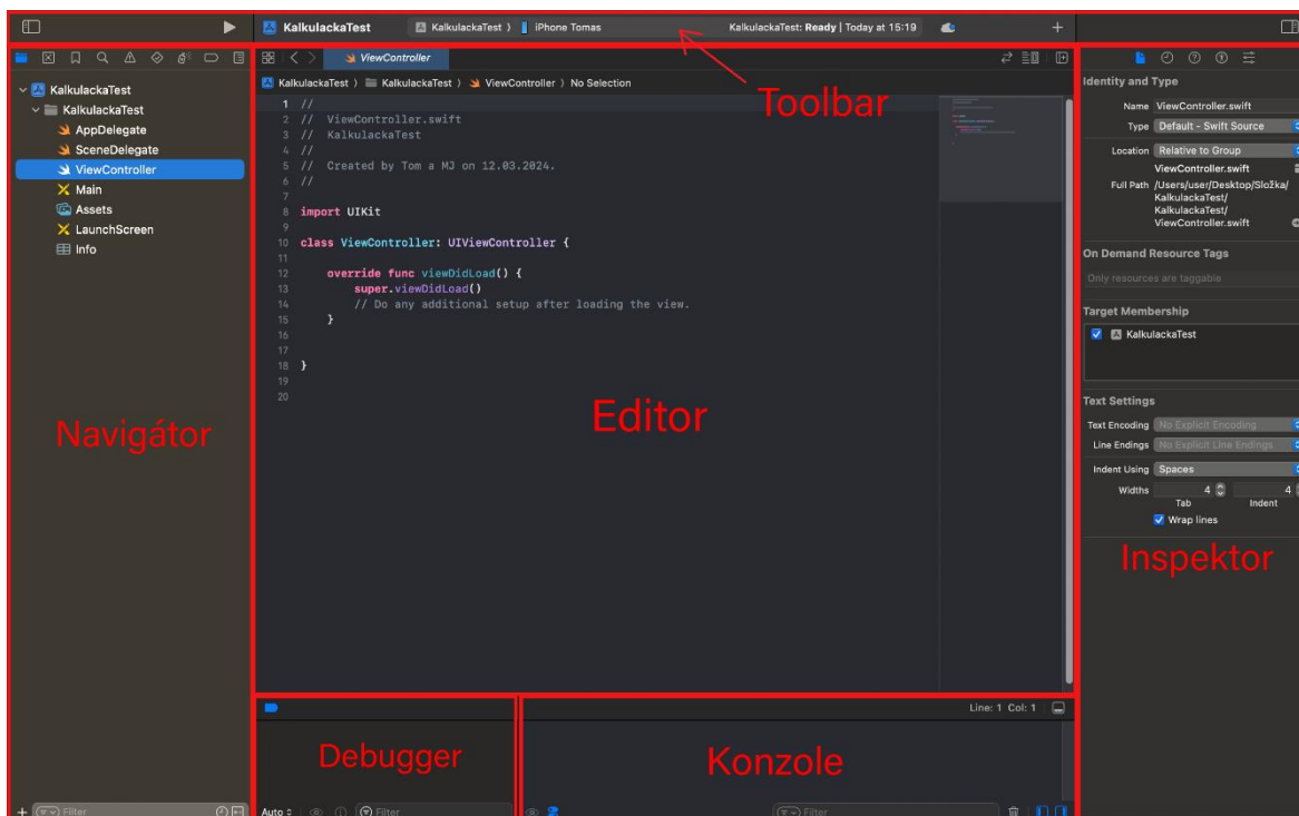
Obrázek 2 - vývojové prostředí
