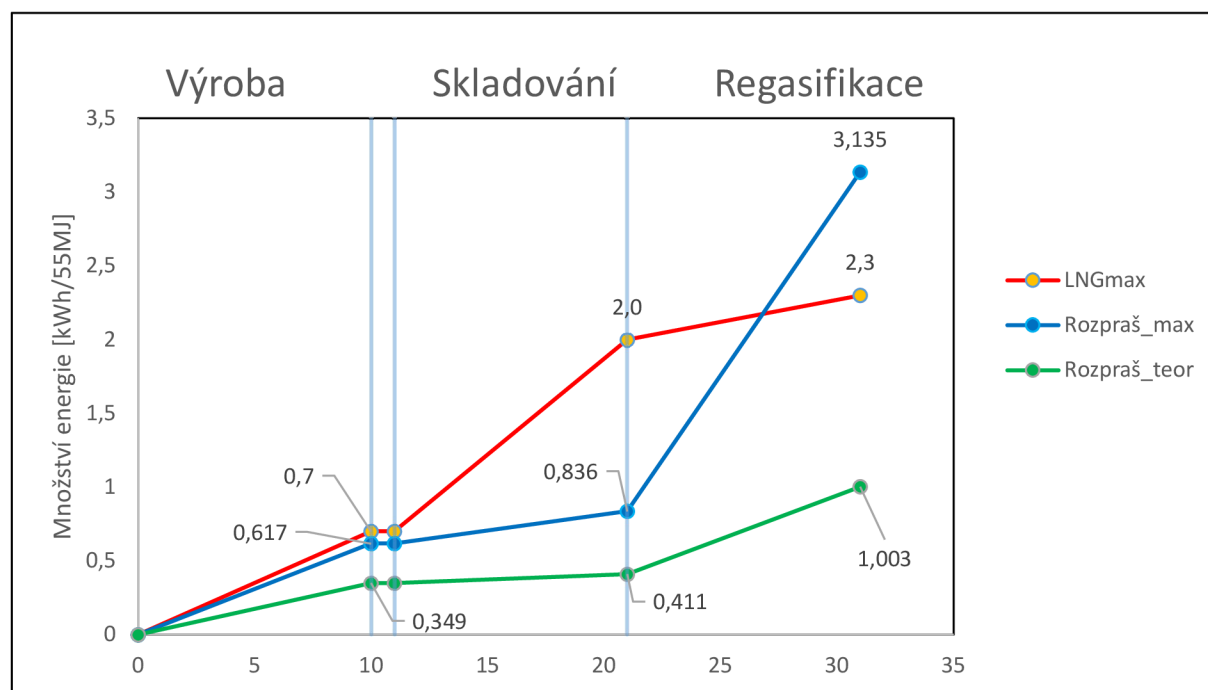
Obrázek 11.2: Graf srovnávající energetickou náročnost výroby, skladování a regasifikace HZP a LNG, vztaženo na 55 MJ
