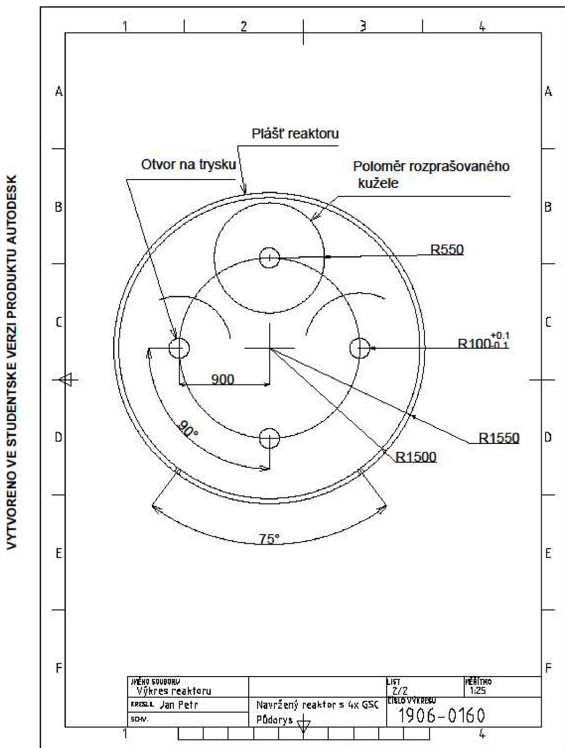
Obrázek 10.5: Přodorys navrženého reaktoru
