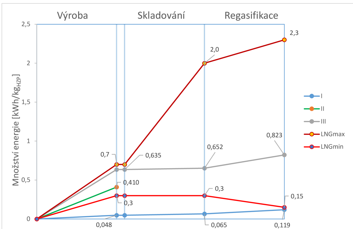
Obrázek 11.1: Graf srovnávající energetickou náročnost výroby, skladování a regasifikace HZP a LNG, vztaheno na 1 kilogram hydrátu zemního plynu
