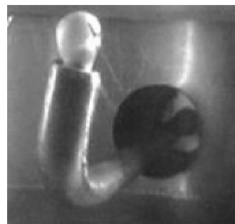
Obrázek 5.5: Hydrát zformovaný na bublině
