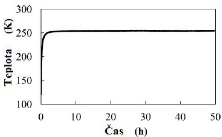
Obrázek 8.9: Nárůst teploty v čase
