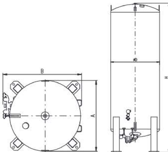
Obrázek 10.8: Vertikální skladovací nádoba VTC52 [58]
