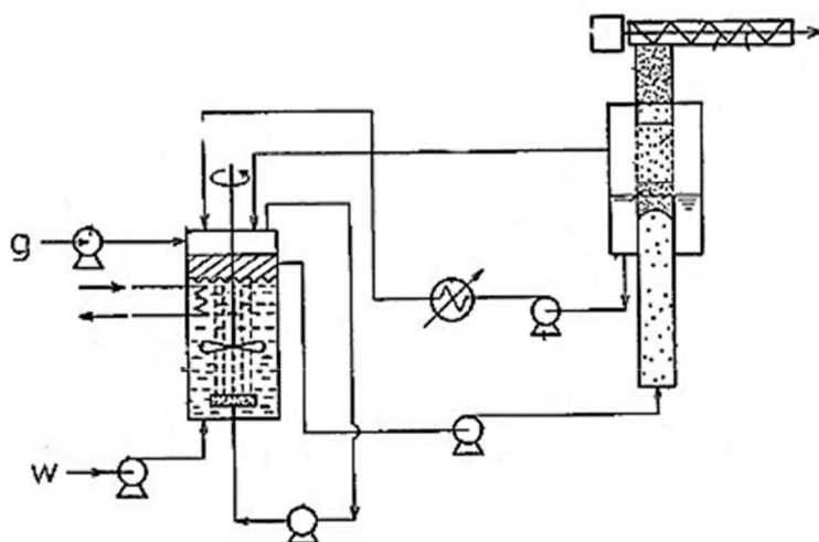
Obrázek 7.1: Proces separace hydrátu gravitační silou [47]
