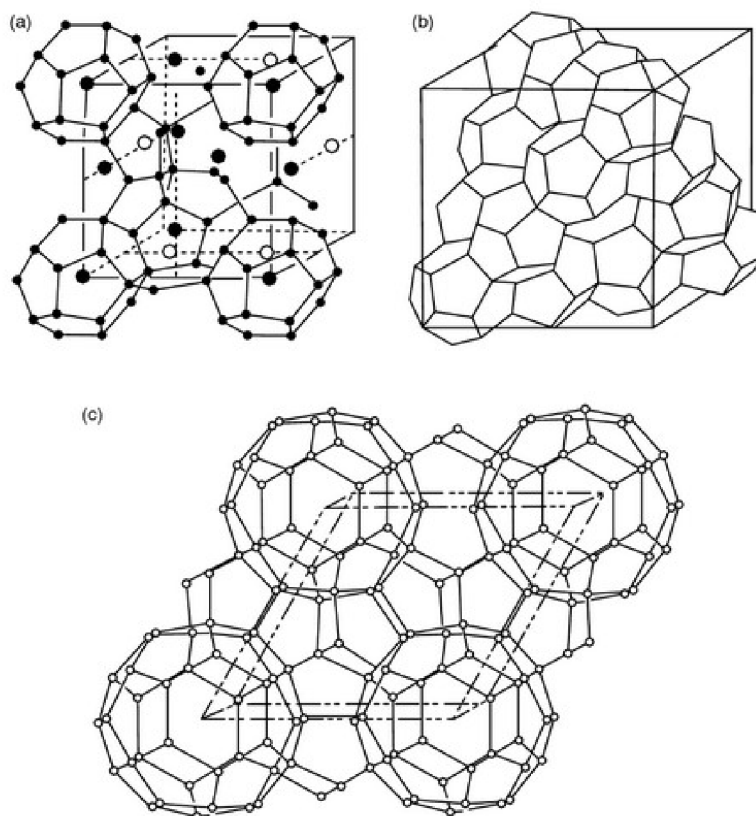
Obrázek 1.6: (a) struktura sI, (b) struktura sII, (c) struktura sH [14]
