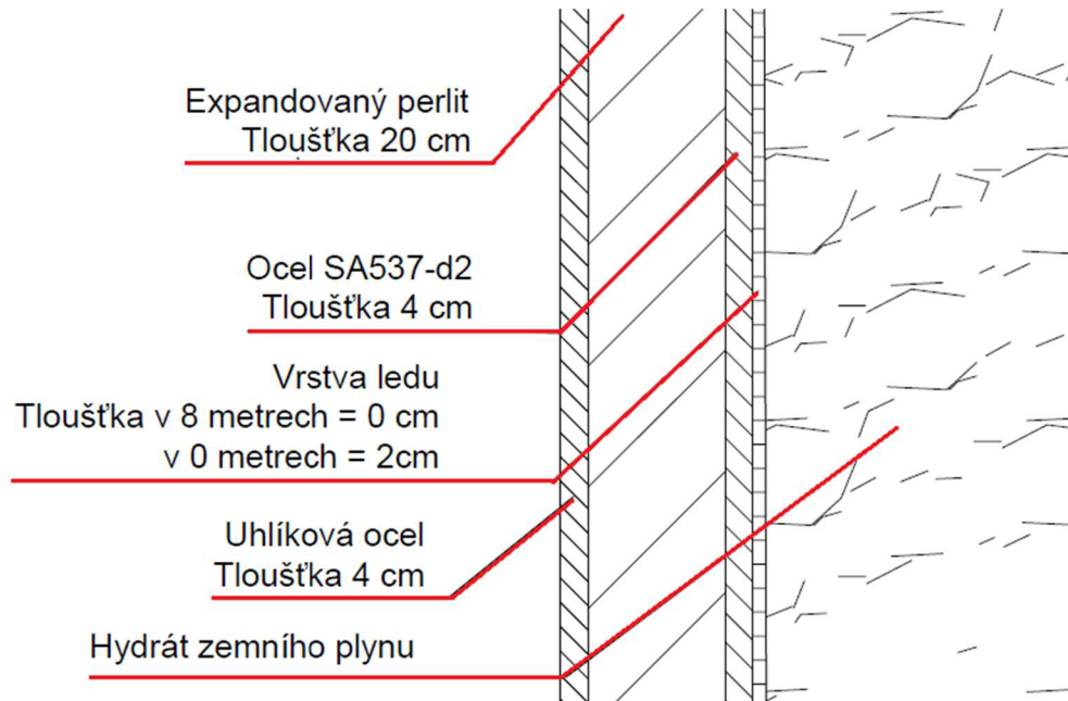
Obrázek 10.10: Detail skladovací nádoby
