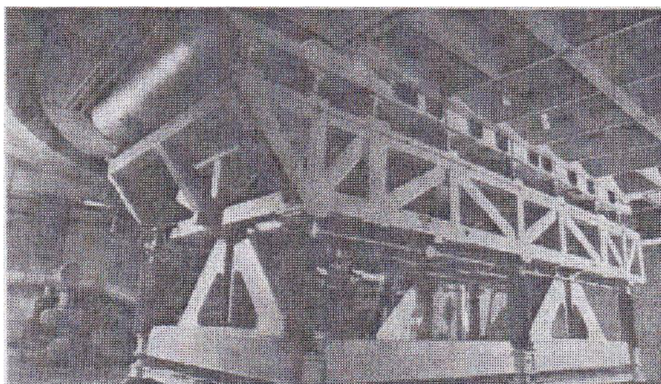
Obr. 9 Pohyblivá pás v aerodynamickom tunely v meste Concord, Severná Karolina[25]
