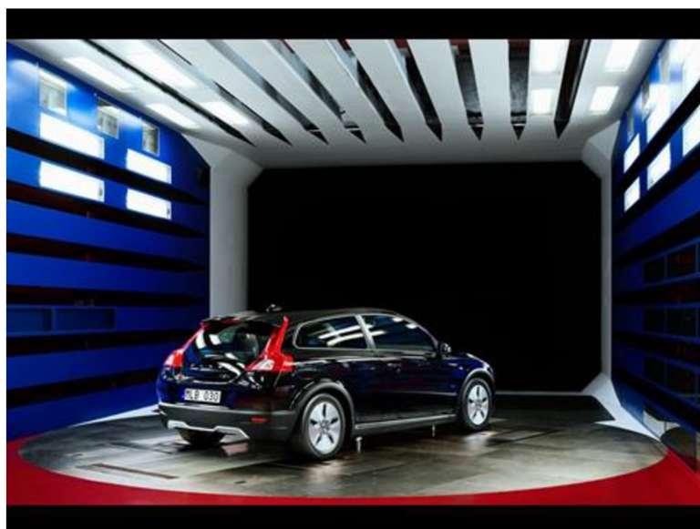
Obr. 24 Natočenie vozidla v aerodynamickom tunely o plus 30 stupňov voči prúdeniu vzduchu[14]
