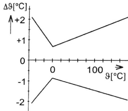
Obrázek 5 Tolerance Ni měřících odporů [2]
