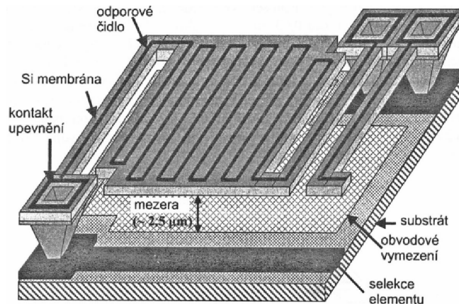
Obrázek 13 Mikrobolometr [2]
