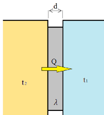
Obrázek 1 Vedení tepla[4]
