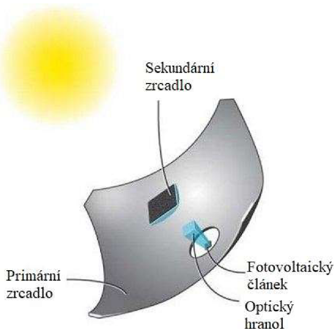
Obrázek 11: Koncentrátor [19]
