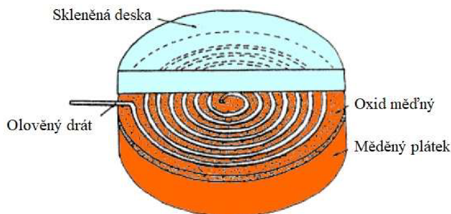
Obrázek 5: Rané Grondahl – Geiger měď-oxid měďné fotovoltaické buňky [3]
