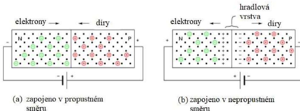
Obrázek 6: P-N přechod [7]
