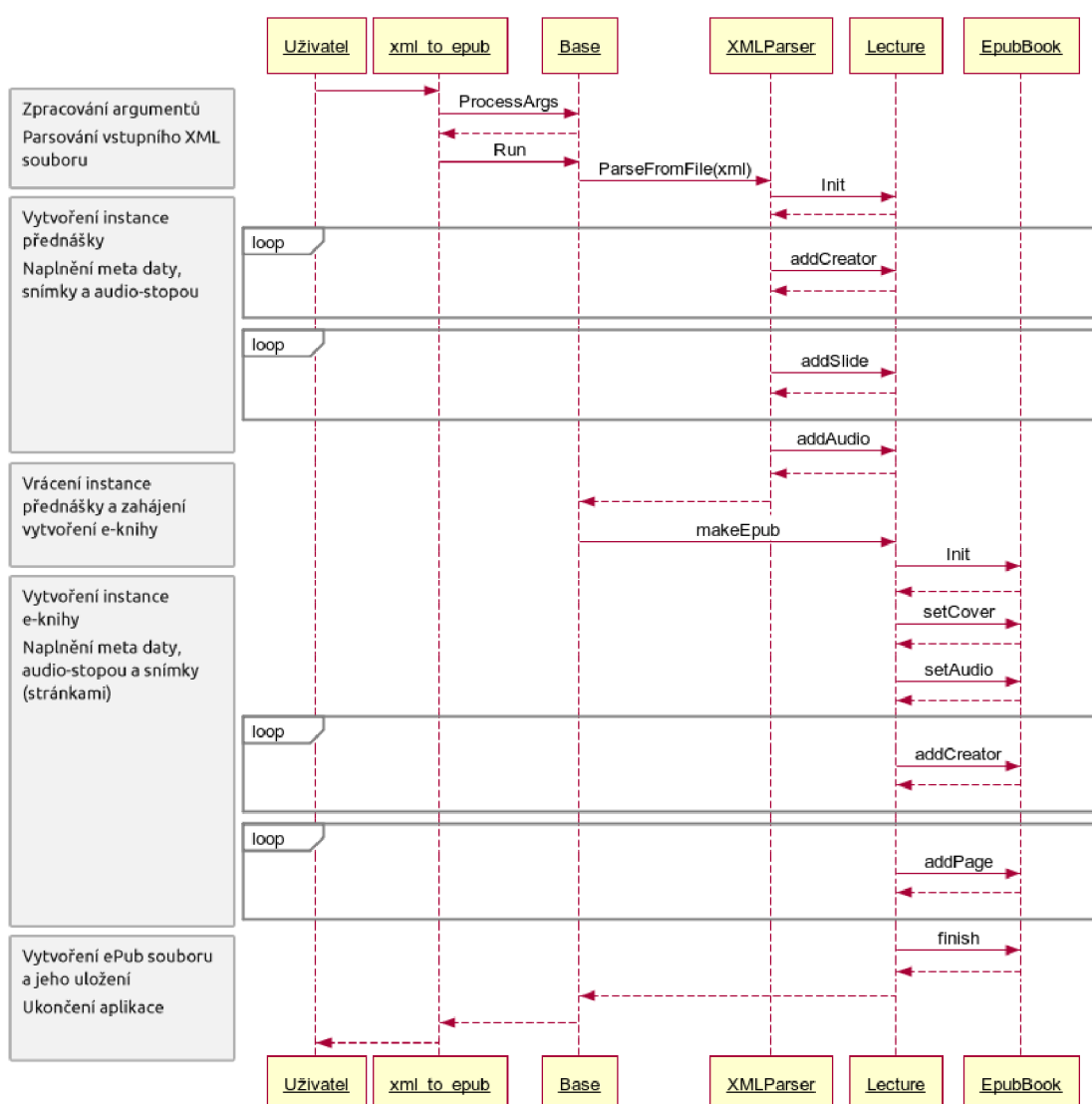
Obrázek B.1: Sekvenční diagram aplikace
