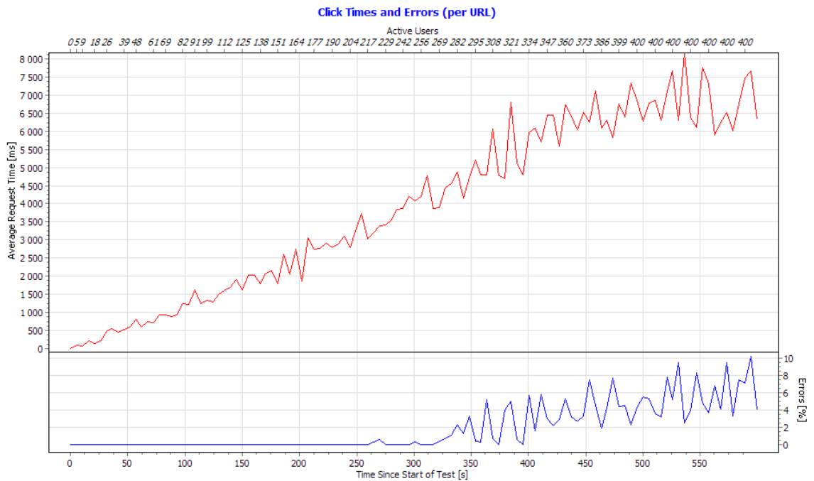
Obrázek 4.1: Požadavek bez autentizace – průměrný čas požadavku a objem chyb
