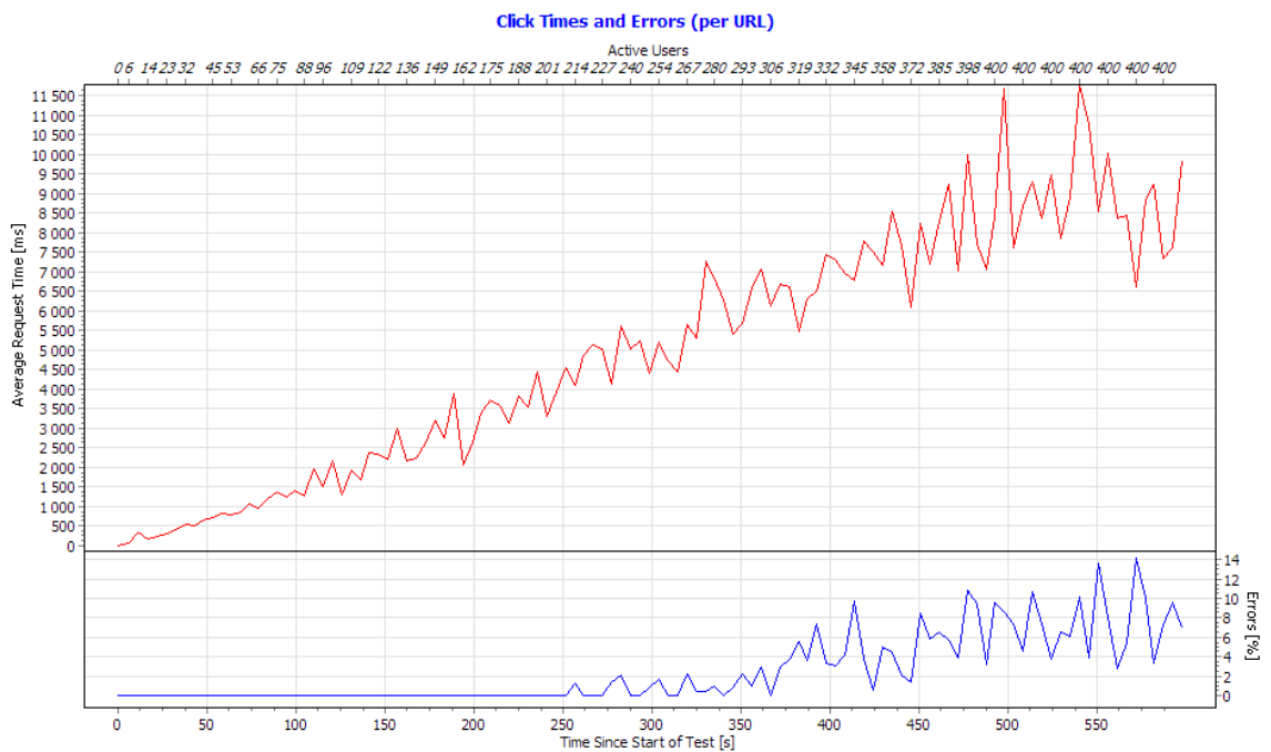
Obrázek 4.2: Autentizovaný požadavek – průměrný čas požadavku a objem chyb
