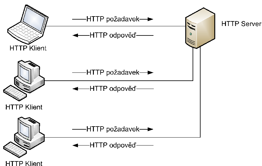
Obrázek 1.1: HTTP protokol
