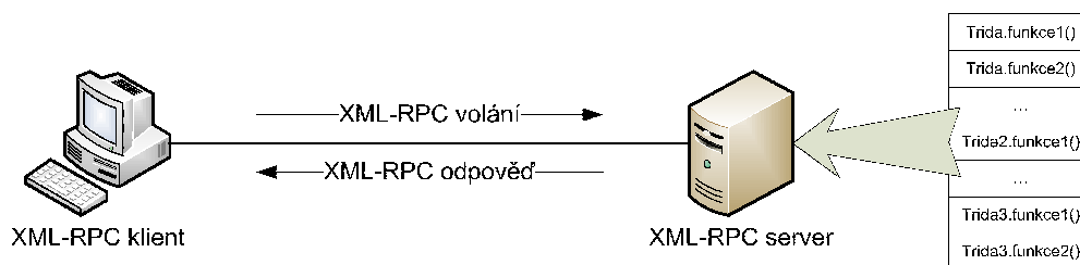
Obrázek 1.2: XML-RPC protokol
