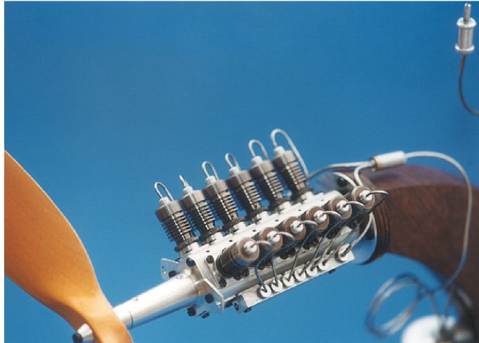
Obrázek 2.6: CO 2 motor
