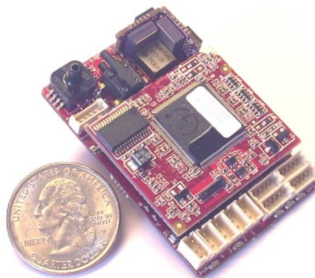
Obrázek 2.5: Kestrel 2.4 Autopilot
