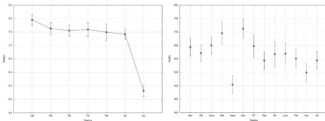
Obr. 17 Vlevo. Analýza variance teplot. CB: České Budějovice; PS: pisek; TB: Tábor; TR: Třeboň; PH: Prachatice; JH: Jindřichův Hradec
