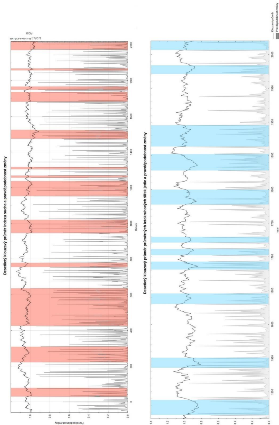
Obr. 28 Vlevo: vyznačení suchých období za posledních 2000 let na základě changepoint analýzy křivky indexů sucha. Data převzata z Büntgen et al. 2021.
