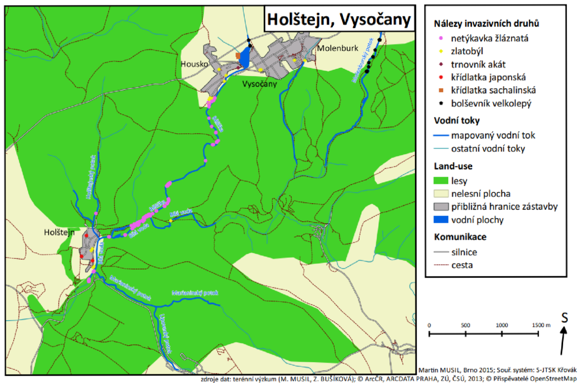
Příloha 4 Mapa vybraných invazivních druhů rostlin okolo vodních toků na hranici Chráněné krajinné oblasti Moravský kras v roce 2015, zdroj: Bušiková & Musil, 2015
