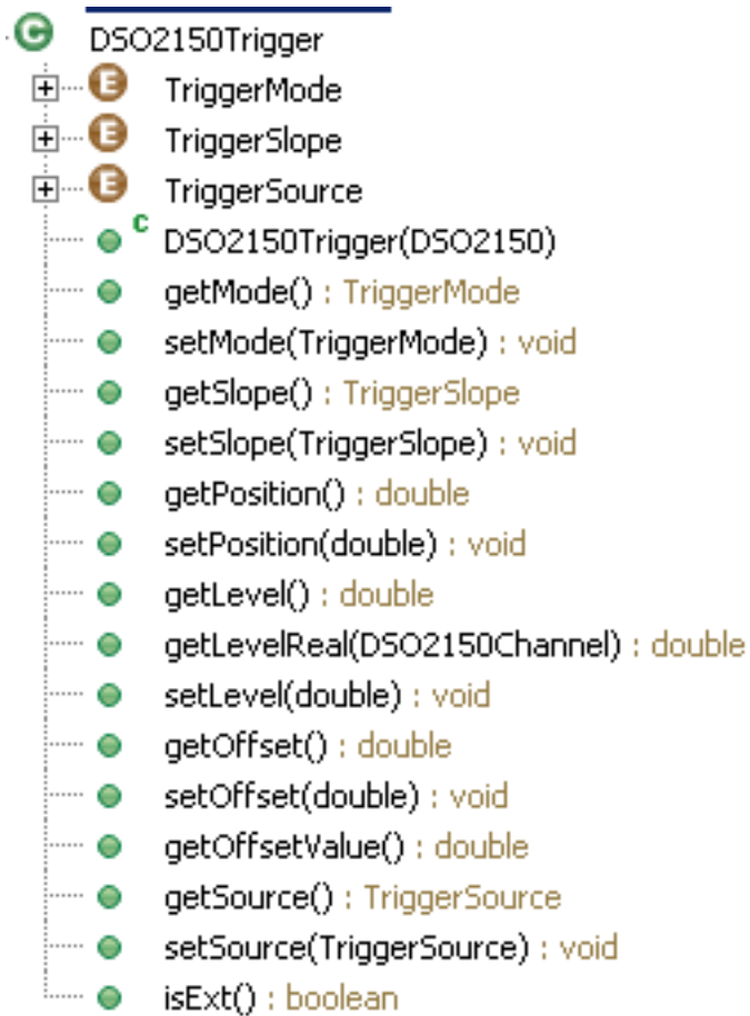
Obr. 5-17 UML diagram třídy DSO2150Trigger
