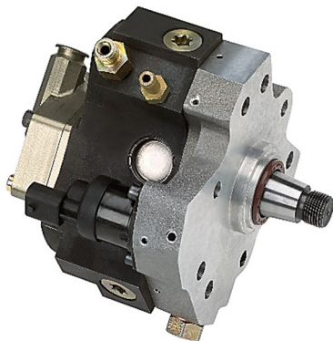
Obr. 3 Čerpadlo CP3 [2]
