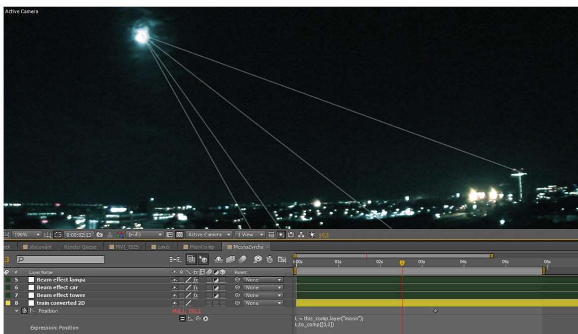
Obrázek 25: Beams efekt
