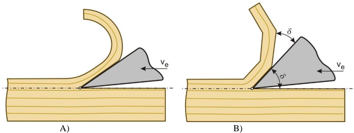
Obrázok č.5 Trieska súvislá špirálová A, trieska časticová mnohouholníková B, zdroj: Siklienka, 2013 (20.2.2023)
