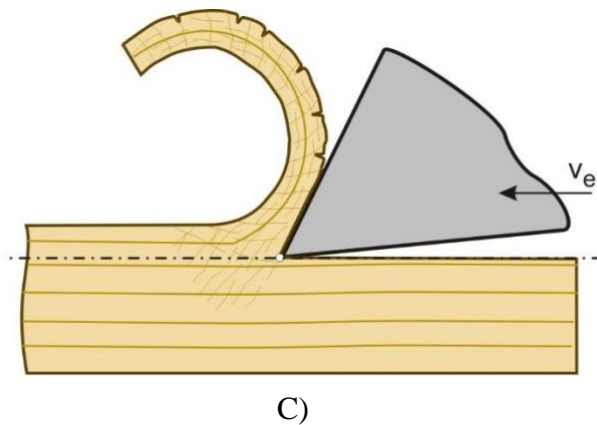
Obrázok č.6 Trieska zhustená súvislá, zdroj: Siklienka, 2013. (20.2.2023)
