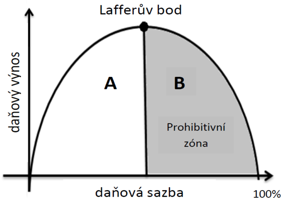
Obrázek 1: Lafferova křivka [9]
