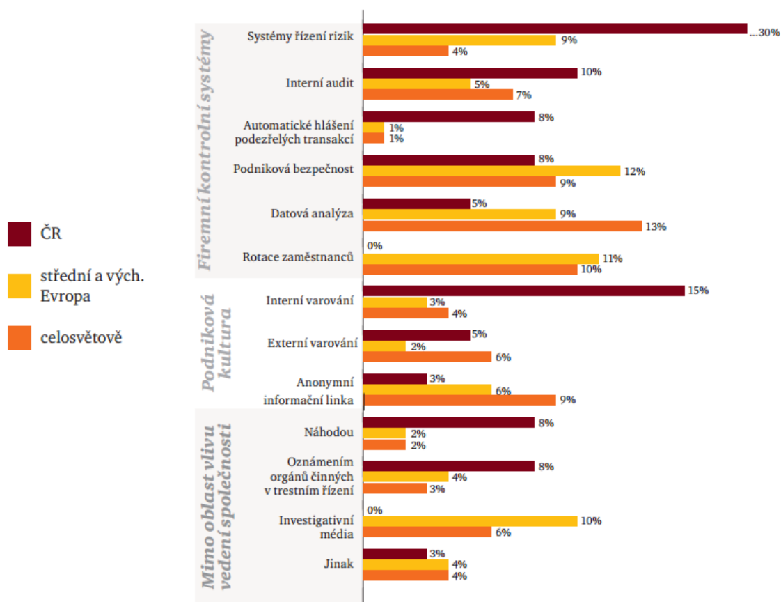
Obrázek 7: Odhalení podvodů [14]
