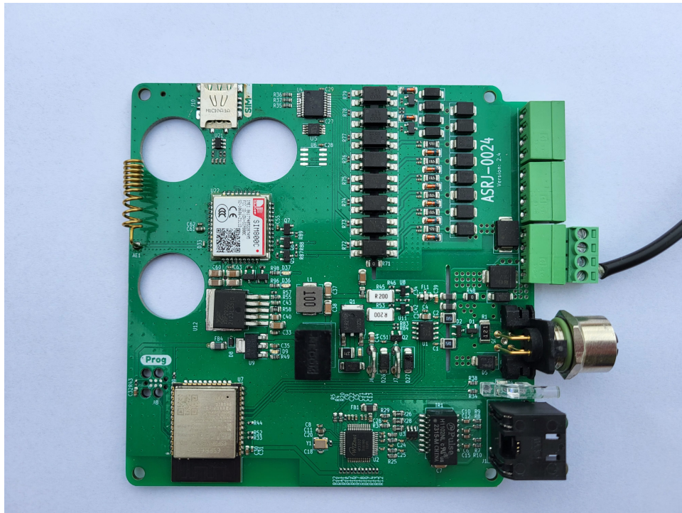
Obr. 3.2: Testovaná DPS
