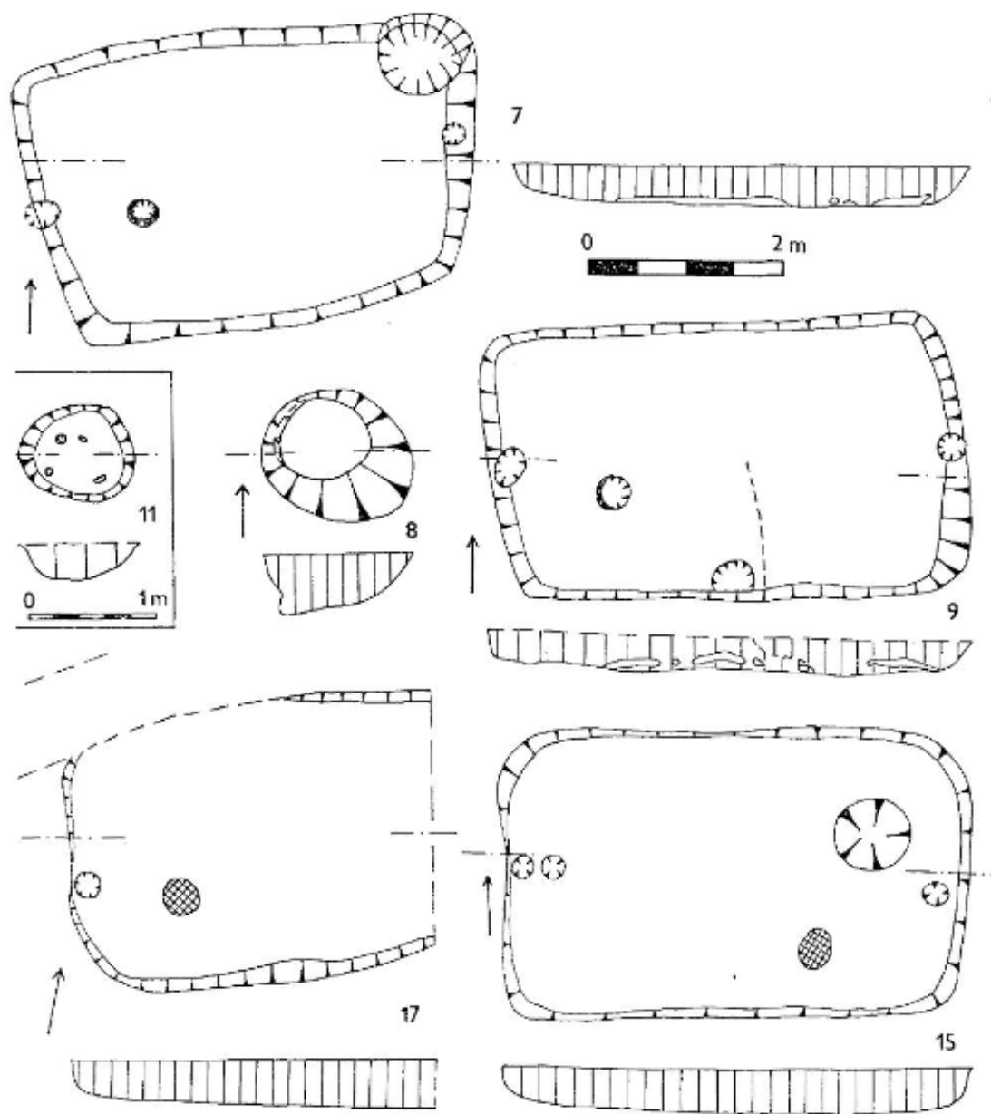
Obr. 32. Břešňany. Zhloubené stavby. Podle Salač 1984, obr. 2.
