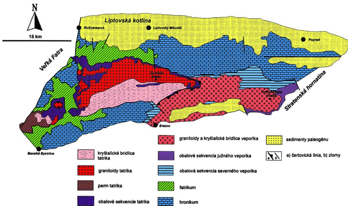
Obr. 2 - Zjednodušená geologická mapa Nízkych Tatier [5]
