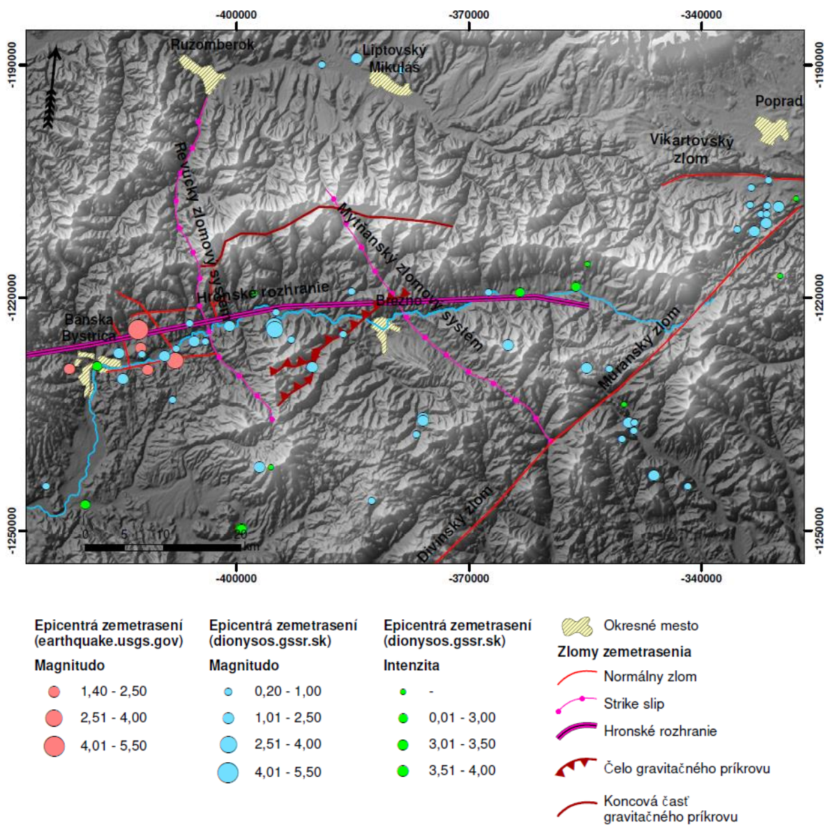
Obr. 13 - Epicentrá zemetrasení v oblasti Nízkych Tatier [24], [25]
