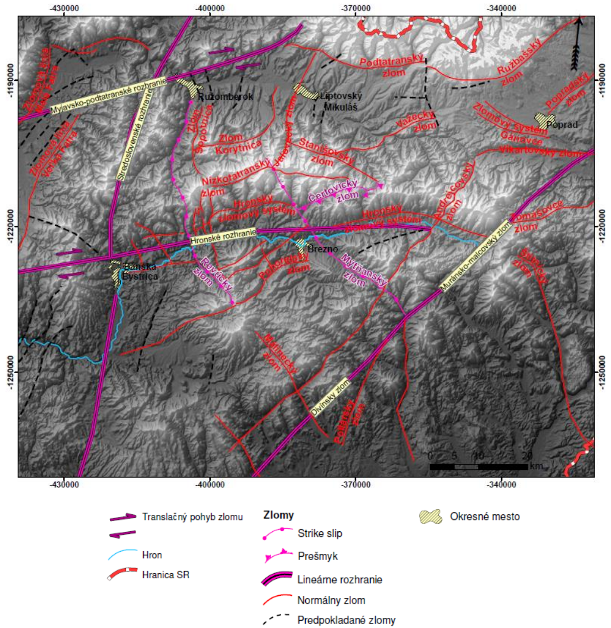
Obr. 5 - Poruchová štruktúra gravitačného príkrovu na južných svahoch Nízke Tatier [22]-upravené
