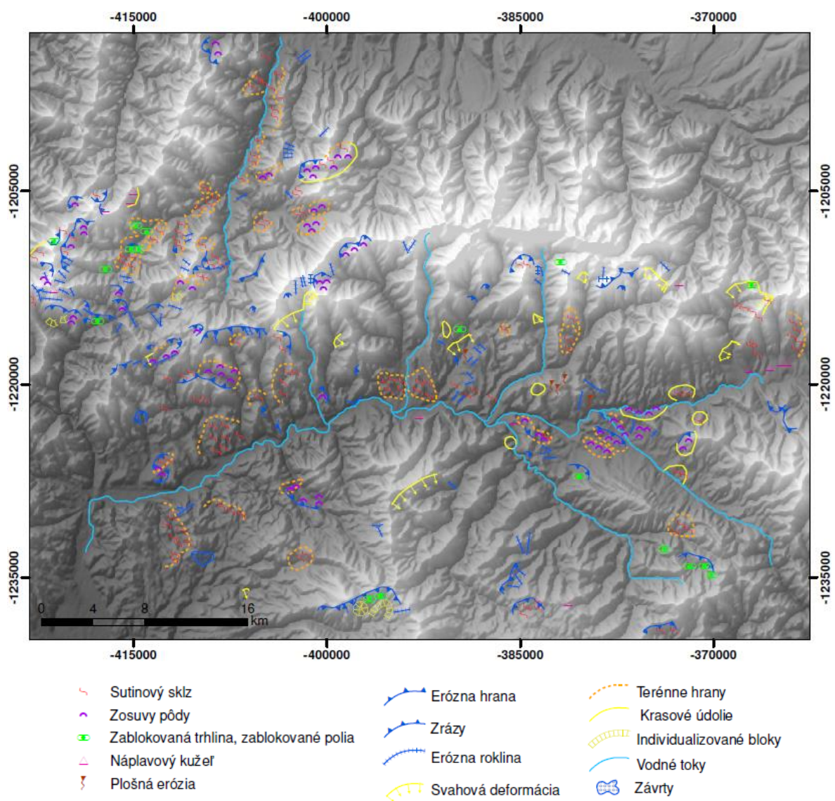
Obr. 15 - Geodynamické javy v Nízkych Tatrách [1]-upravené
