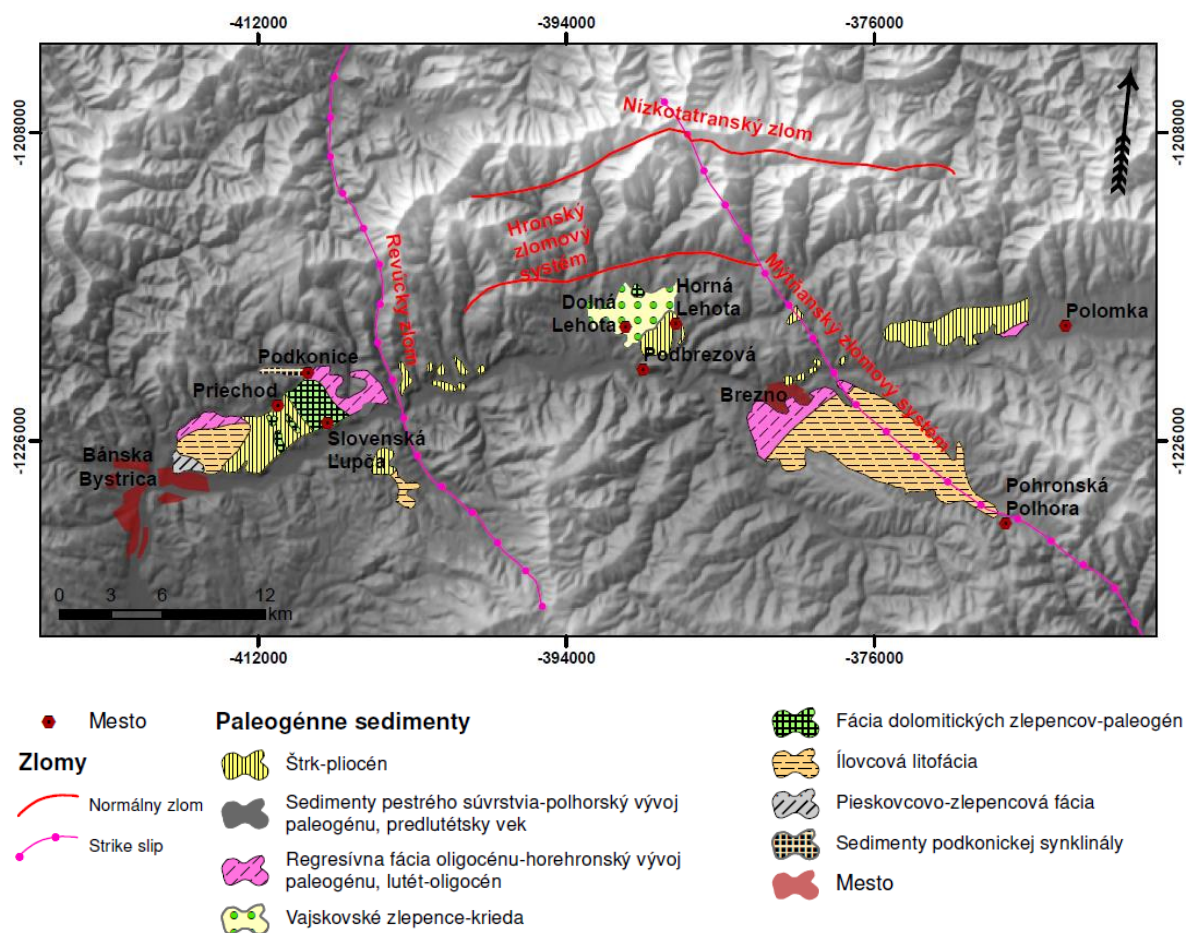
Obr. 4 - Paleogénne sedimenty v oblasti Nízkyh Tatier [2]-upravené
