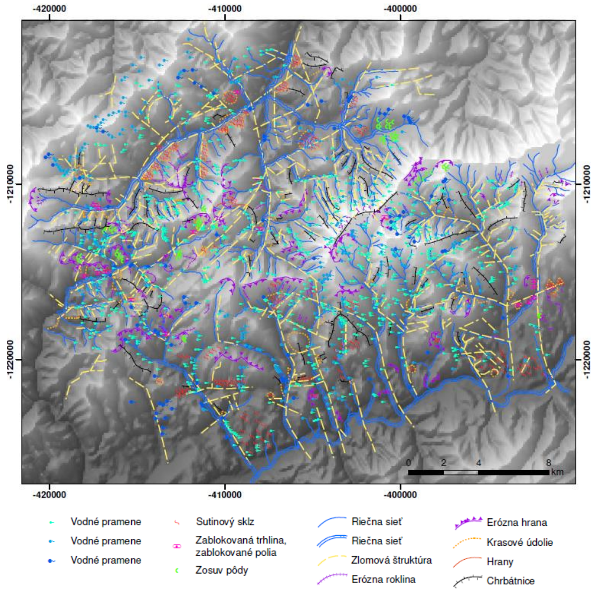
Obr. 16 - Geodynamické javy a obraz vodných tokov a prameňov v Ďumbierskej časti Nízkych Tatier
