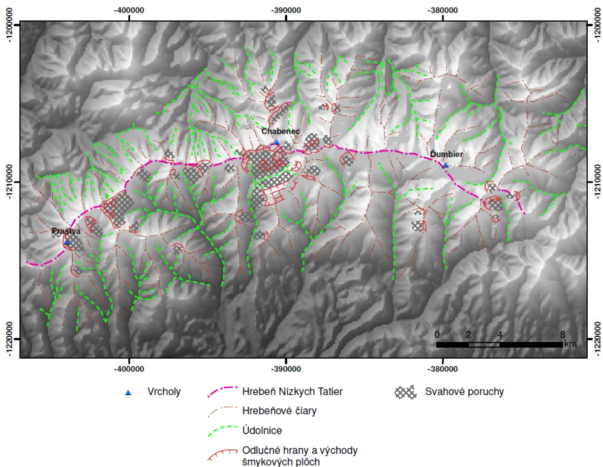
Obr. 14 - Hlbinné svahové poruchy na hrebeňoch Prašivej, Chabence a Ďumbiera [26]-upravené
