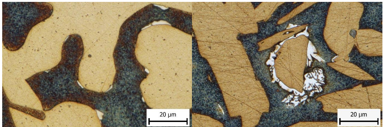
Obr. 4.3 Mikrostruktura intermetalických fází ze vzorku ŘO_2.
