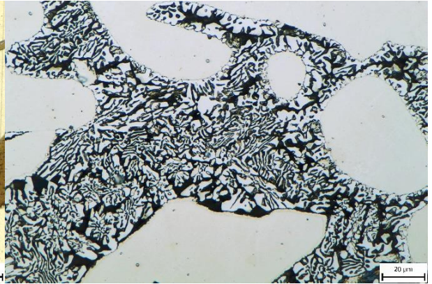
Obr. 2.11. Mikrostruktura (žiháno při 800 °C 50 h, SM).
