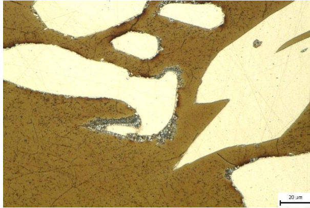
Obr. 2.10 Mikrostruktura (žiháno při 800 °C 1 h, SM).
