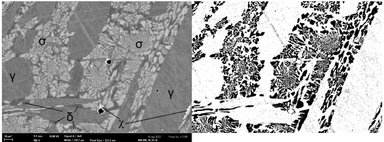
Obr. 3.1 Mikrostruktura (žíháno při 800 °C 50h, SEM).
