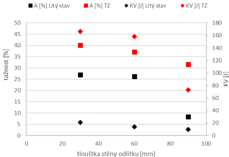
Obr. 1 Vliv tloušťky stěny na tažnost a nárazovou práci oceli A890 GR4A v litém stavu a po rozpouštěcím žíhání [14].
