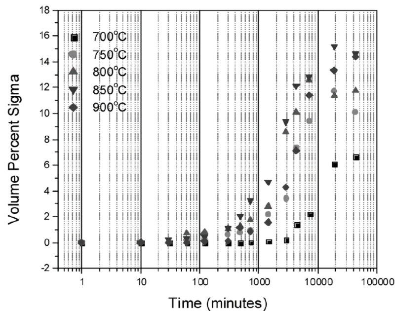
Obr. 3.7 Transformační diagram lité duplexní oceli CD3MN [32].
