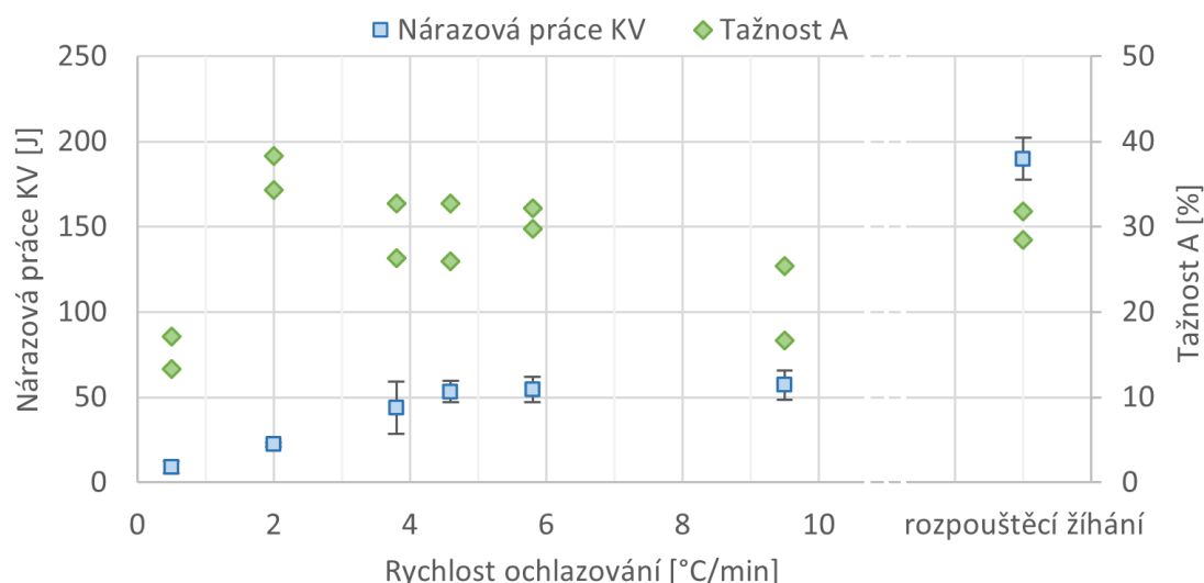
Obr. 4.1 Nárazová práce a tažnost v závislosti na rychlosti ochlazování.
