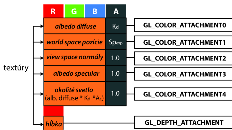
Obr. 6.1: Implementovaný G-buffer. K_d reprezentuje odrazivý koeficient materiálu a S_{exp} ( shininess ) lesklosť povrchu, popísané v kapitole 3.1
