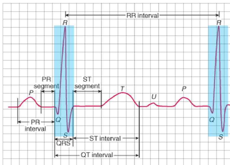
Obrázok 6:QRS komplex [2]
