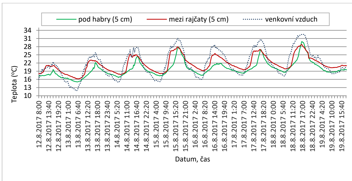
Obr. 4.29 - Průběh teplot v substrátu vegetační střešky v hloubce 5 cm pod habry a mezi rajčaty ve srovnání s teplotami vzduchu (12.8.-19.8.2017)
