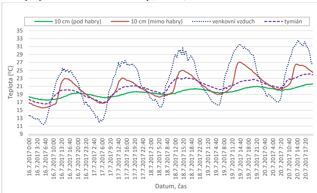
Obr. 4.27- Průběh teplot v substrátu (senzor (1) - 10 cm pod habry, senzor(2)- 10 cm mimo habry, teplotní čidlo (3) umístěné těsně pod povrchem v tymiánu) a průběh teplot venkovního vzduchu (16.7-20.7.2017)
