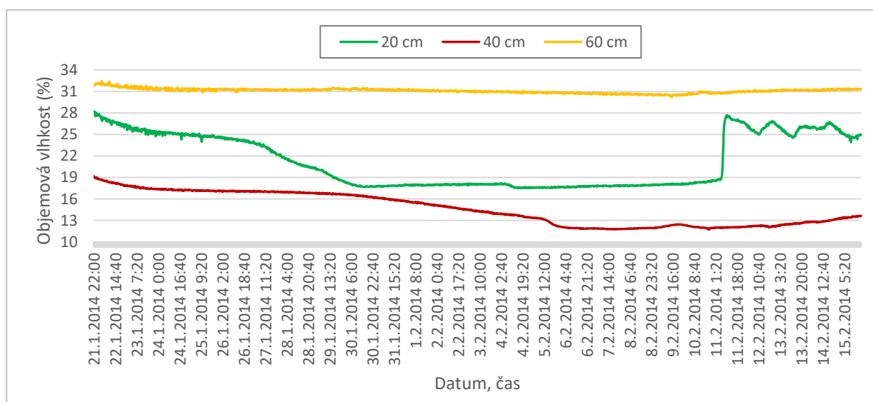
Obr. 4.4 - Objemová vlhkost (v %) v substrátu intenzivní vegetační střechy v hloubkách 20, 40 a 60 cm v zimním období od 21.1. do 15.2.2014
