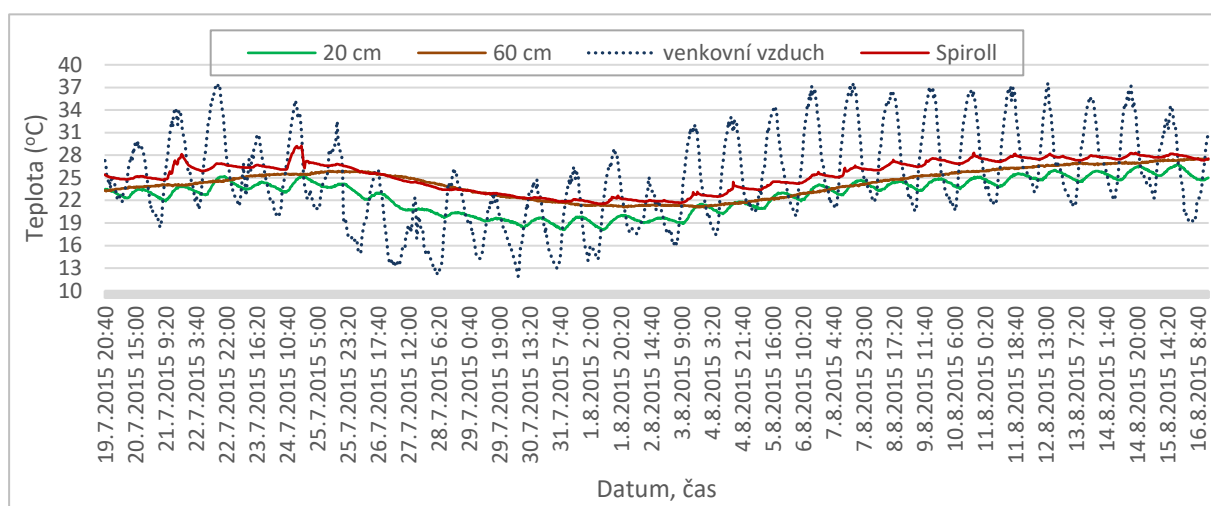
Obr. 4.19- Průběh teplot na stropě zahradního domku v porovnání s teplotami v substrátu vegetační střechy a s teplotami venkovního vzduchu naměřenými meteostanicí Em50 (19.7.-16.8.2015)
