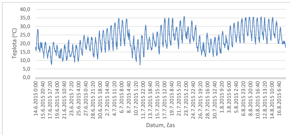
Obr. 4.15- Průběh teplot venkovního vzduchu v období od 14.6. do 17.8.2015 (zdroj: data ČHMÚ, meteorostanice (B2BTUR01) Brno-Tuřany)
