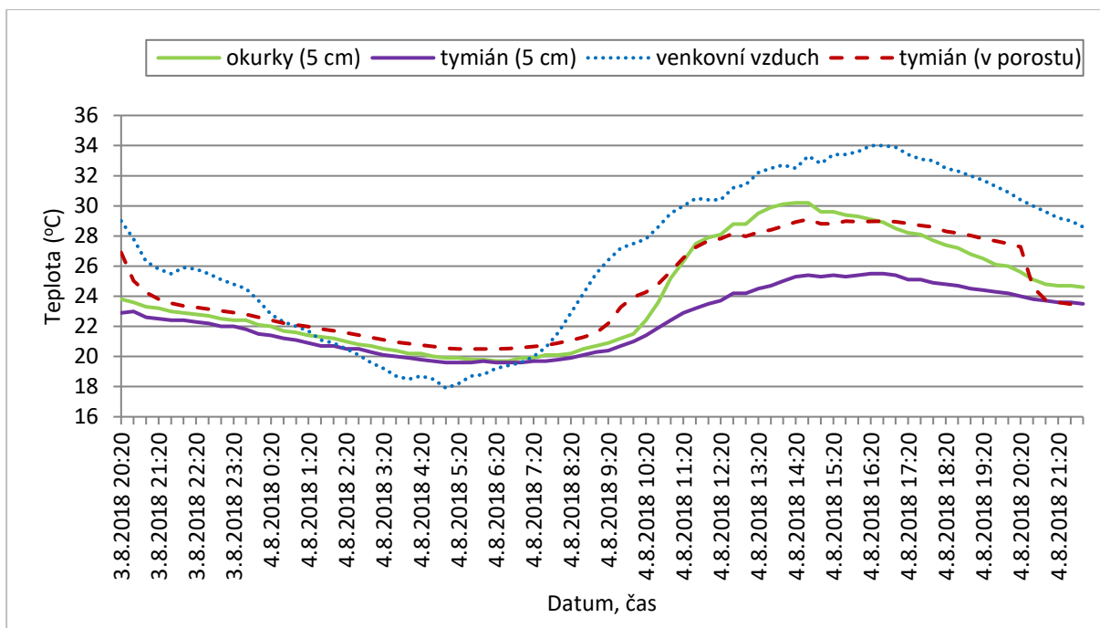
Obr. 4.34- Průběh teplot v substrátu (5 cm - okurky, 5 cm – tymián), ve srovnání s teplotou venkovního vzduchu a naměřenou teplotou v porostu tymiánu (teplotní čidlo (3) připojené k meteostanici Em50)
