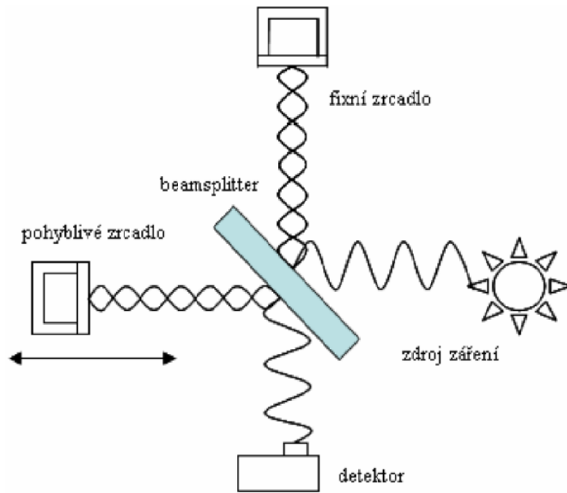
Obrázek 9 Michelsonův interferometr [38]
