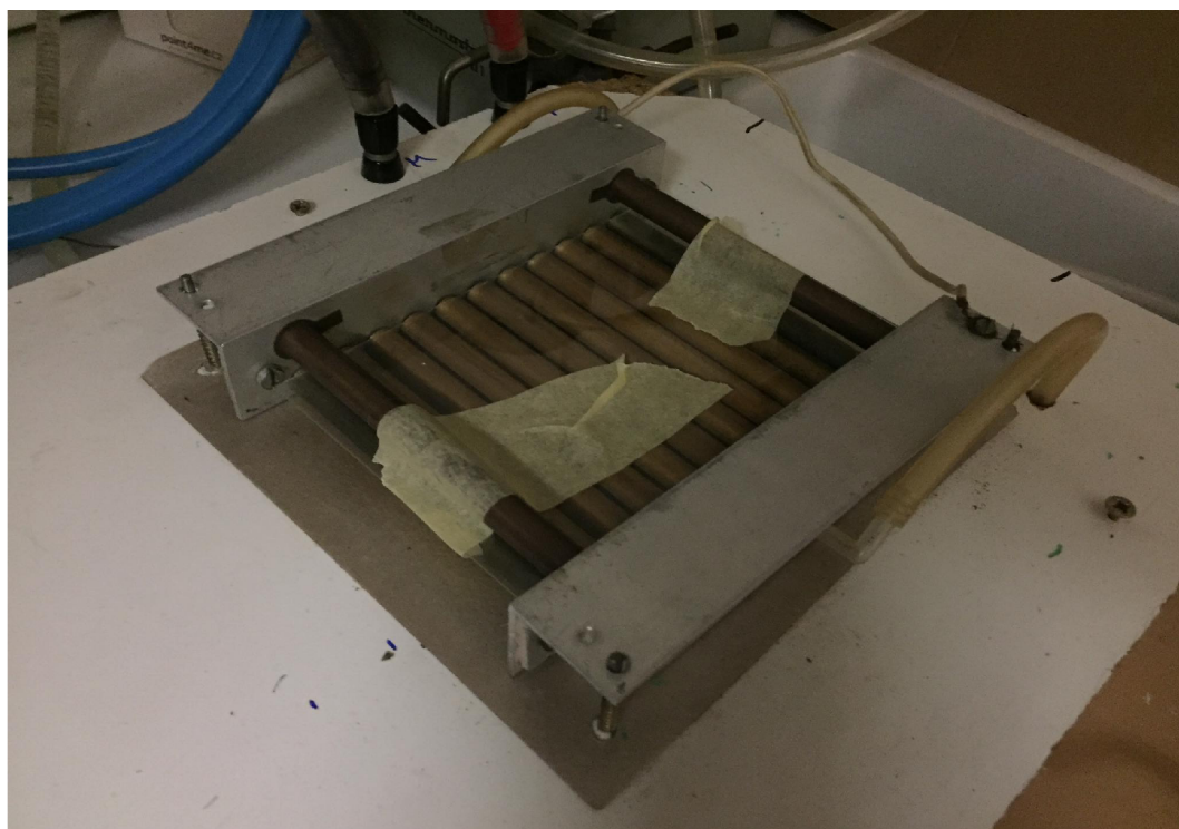
Obrázek 14 Použitý elektrodotý systém v povrchovém uspořádání
