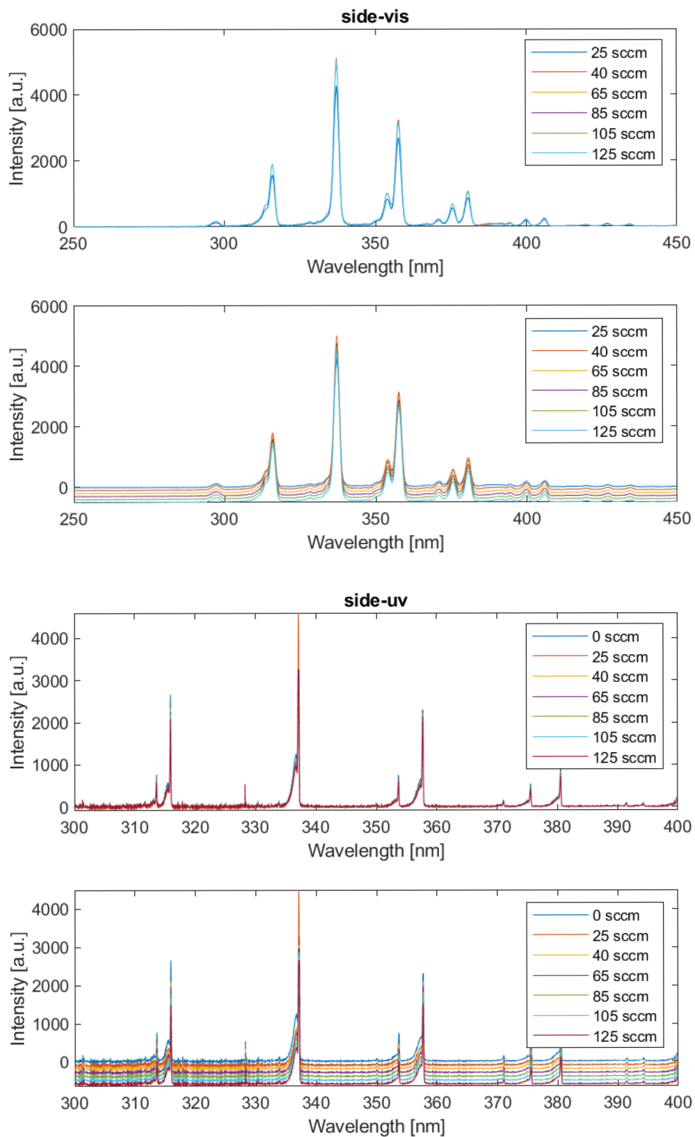
Obrázek 17 Závislost intenzity signálu na vlnové délce při SIDE měření ve viditelné a ultrafialové oblasti
