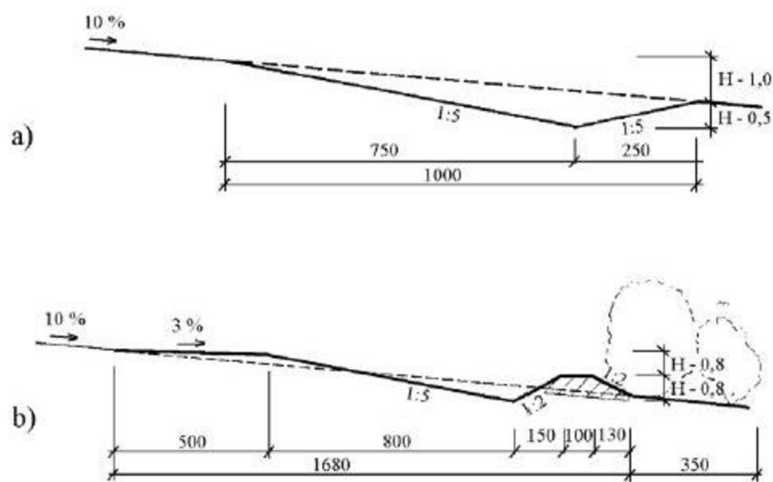
Obr. 2.1 a) průleh, b) průleh s přidanou hrázkou [14]
