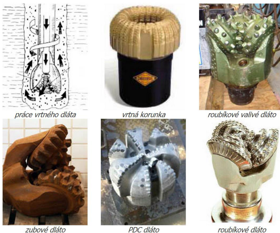
Obr. 6.4 Vrtná dláta [13]
