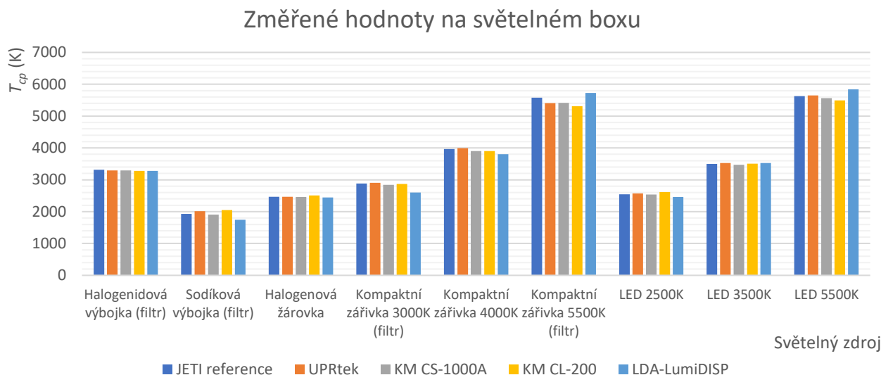
Obr. 51 Změřené hodnoty T_{cp} na světelném boxu
