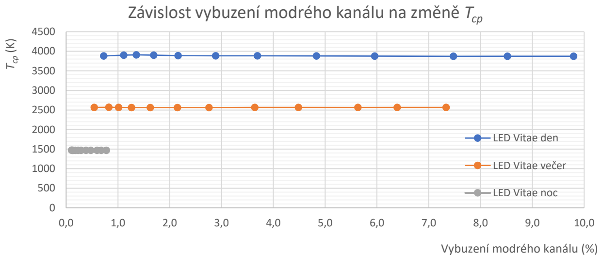
Obr. 82 Závislost vybuzení modrého kanálu na změně T_{cp}
