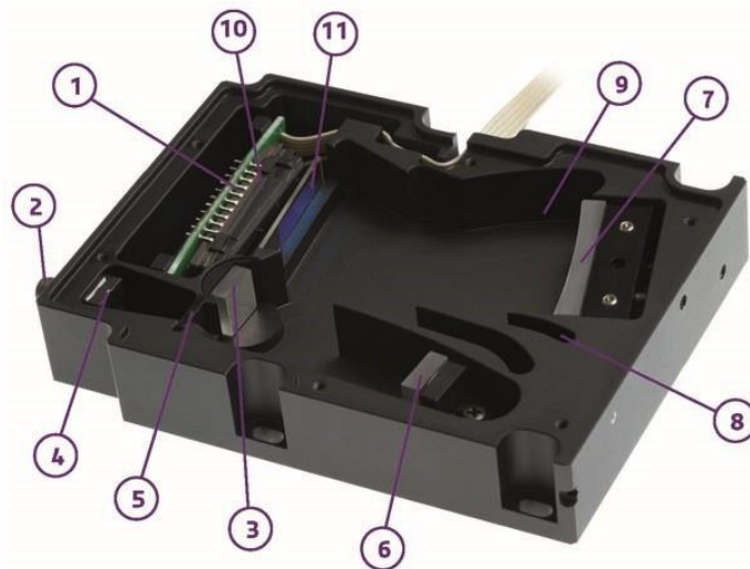
Avaspec-ULS Složení optické lavice: Symetrické uspořádání
