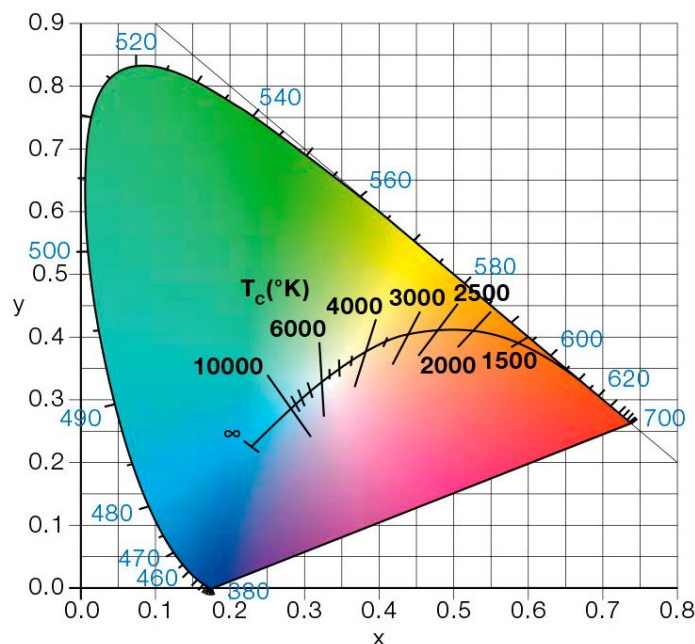
Obr. 8 Diagram chromatičnosti CIE ( x, y ) s vyznačenou křivkou teplotního zářiče [18]
