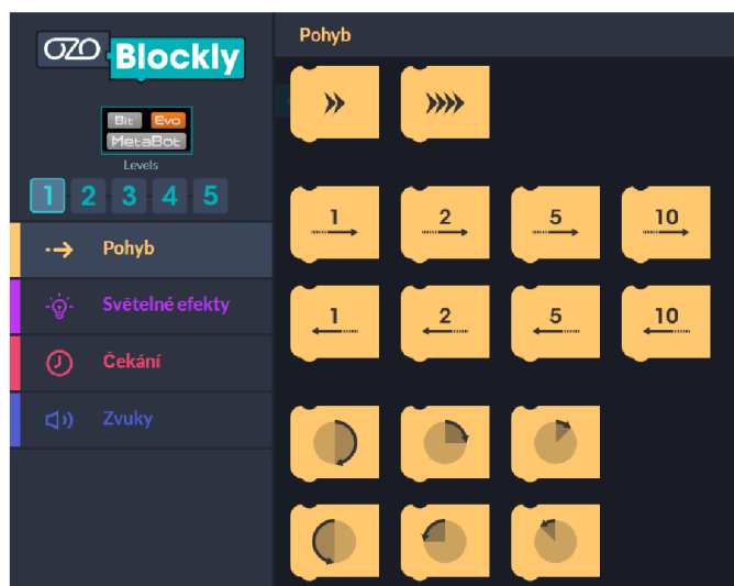
Obrázek 5: Úroveň 1 - Nováček
