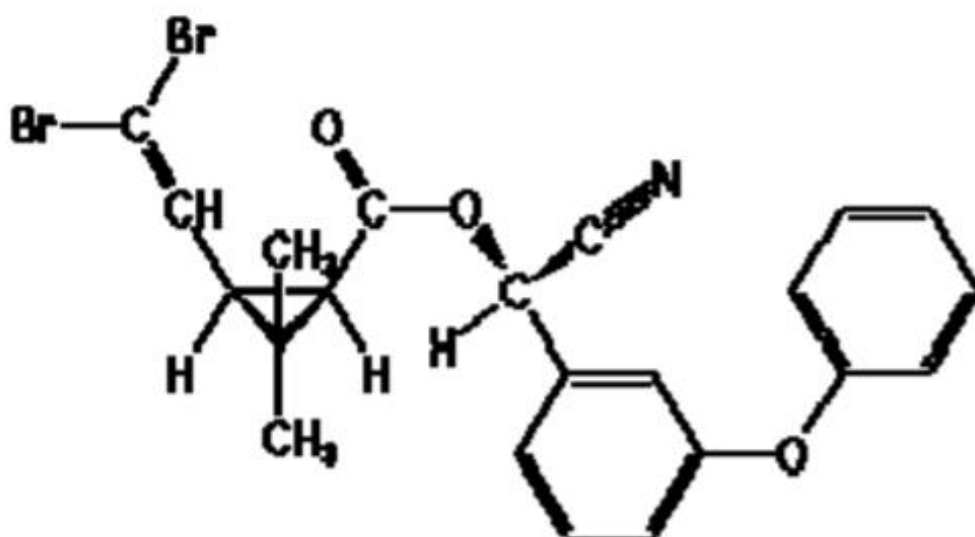
Příloha 19 – strukturální vzorec Deltamethrin (EFSA 2010)
