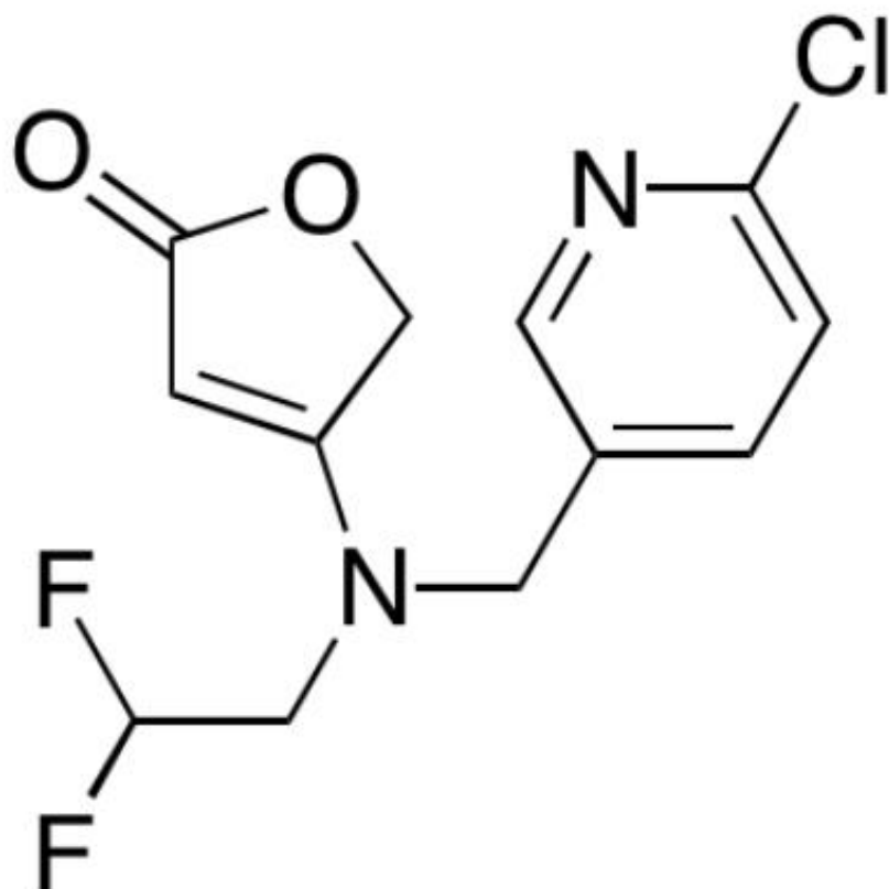
Příloha 18 – strukturální vzorec Flupyradifuron (Nauen et al. 2014)
